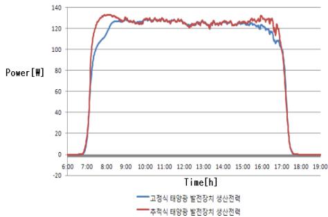
[그림 7] 맑은 날의 출력전력 그래프
