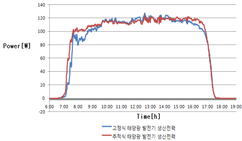
[그림 8] 흐린 날의 출력전력 그래프
