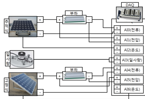
[그림 5] 모니터링 구성도
