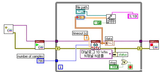
[그림 6] 데이터취득 프로그램
