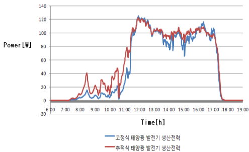
[그림 9] 비오고 흐린 날의 출력전력 그래프
