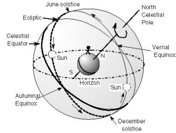
[그림 2] 천구의 정의
