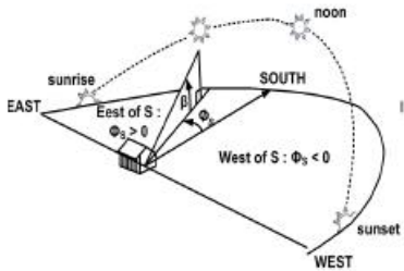
[그림 1] 태양의 고도각 및 방위각
