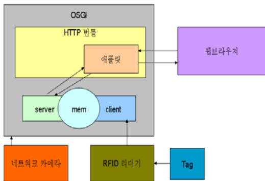
(그림 7) RFID 시스템 구성도
