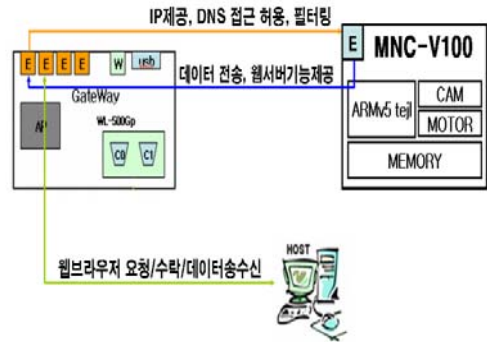
(그림 6) 게이트웨이와 카메라 간 흐름도
