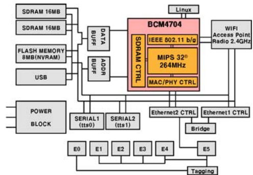
(그림 4) 게이트웨이 블록 다이어그램
