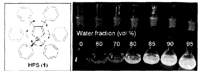
그림 10. (좌측) 화학 구조 (우측) 비용매인 물의 첨가량에 따른 hexaphenylsilole 용액의 형광변화 사진.
