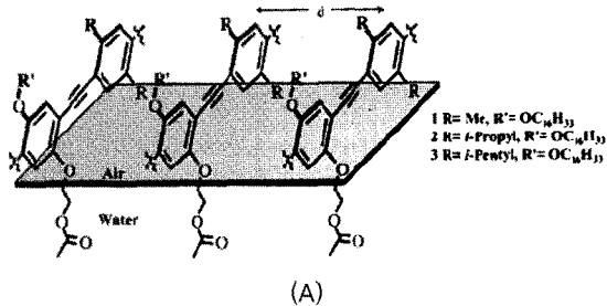
그림 1. 형광 공역 고분자의 conformation 변화에 따른 발광파장의 변화. 뒤틀림 구조에 의한 공역 길이 저하에 따른 발광파장의 단파장 이동과 평면화에 기인한 공역길이 증대에 따른 발광파장의 장파장 이동현상 발생. 3
