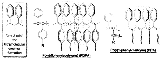
그림 8. 이치환형 아세틸렌폴리머의 구조와 n=3 의 법칙에 따른 분자내 엑시머의 형태.
