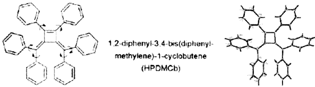
그림 12. 결정구조적으로 투폴드 대칭(twofold symmetry)구조를 가지는 분자.
