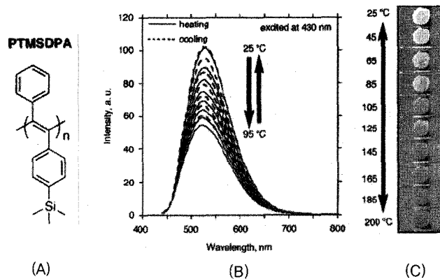
그림 3. (A) 이치환형 아세틸렌 폴리머의 화학적 구조와 (B) 온도에 따른 형광강도의 변화 모습. (C) 온도에 따른 공역 고분자의 형광 이미지.
