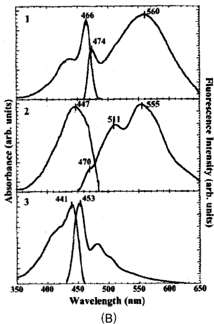
그림 2. 분자간 거리에 따른 광 물리적 특성의 변화. (A) Langmuir-Brodget 방법으로 분자간 거리를 조절. (B) 분자간 거리가 가까워질수록 형광의 장파장 이동과 형광효율이 낮아지는 현상을 보인다.
