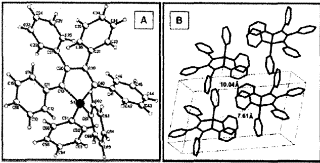
그림 17. (A) CIE 현상을 보이는 hexaphenylisilole의 구조를 ORTEP로 그린 모습. (B) Hexaphenylisilole의 패킹 다이어그램.
