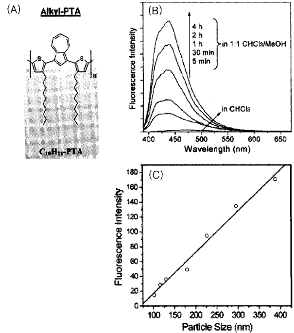
그림 16. (A) Poly{1,3-bis[2-(3- n -decylthienyl)]azulene} ( C_{10}H_{21} -PTA)의 화학적 구조식과 chloroform과 methanol의 1:1 혼합용액안에서 시간에 따른 (B)형광 스펙트럼의 변화. (C) 나노입자크기의 증대와 형광강도의 관계.
