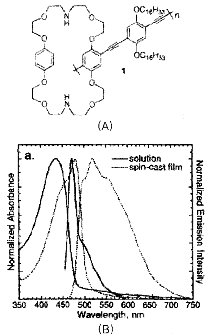
그림 6. (A) Alkoxy-PPE의 화학구조, (B) 용액상과 스핀코팅한 필름 각각의 UV-vis 흡수 스펙트럼과 형광 방출 스펙트럼.
