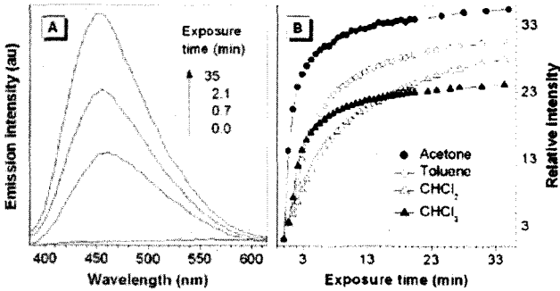
그림 18. (A) 석영위에 코팅된 CIEE 현상을 나타내는 공역분자의 acetone 증기에 노출된 시간에 따른 형광 방출 스펙트럼의 변화. (B) 다양한 용매 증기에 따른 노출시간당 형광강도의 변화.
