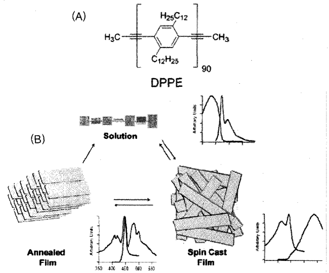
그림 19. (A) didodecyl-PPE의 화학적구조와 (B) 고체상과 용액상에서의 광학거동.
