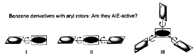
그림 11. Benzene 중심(검은색 타원)에 aryl 치환기를 하나 (I), 둘 (II) 셋(III) 가지는 형광 분자.
