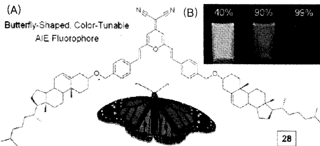
그림 13. (A) 나비모양의 AIE 형광체의 나노회합체. (B) THF-물 혼합용액에서 물의 함량이 40, 90, 99%로 변함에 따라 발광색이 녹색 황색 적색으로 변하는 모습.
