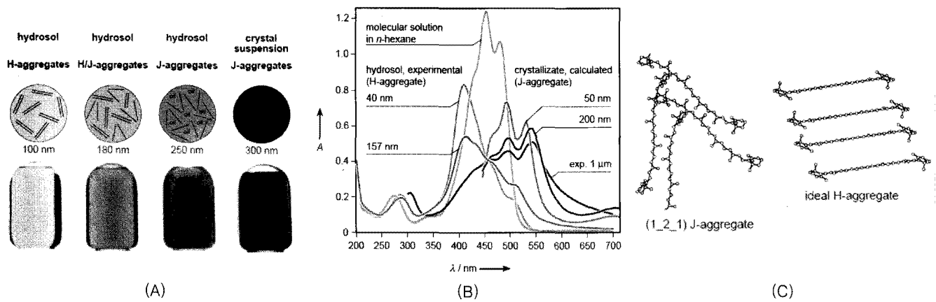
그림 5. (A) \beta -carotene hydrocol의 회합체 구조와 입자크기에 따른 색변화와 (B) 자외-가시광 흡수 스펙트럼의 변화. (C) J-type과 H-type의 회합구조체의 모식도.
