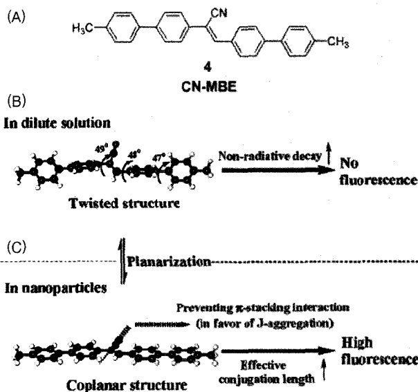
그림 4. (A) AIEE특성을 가지는 CN-MBE의 화학적 구조와 (B) 희박용액 안에서의 CN-MBE의 뒤틀려 있는 모습. (C) CN-MBE 분자들이 서로 회합됨에 따라 서로간의 충진력에 기인해 공평면 구조를 가지는 모습.
