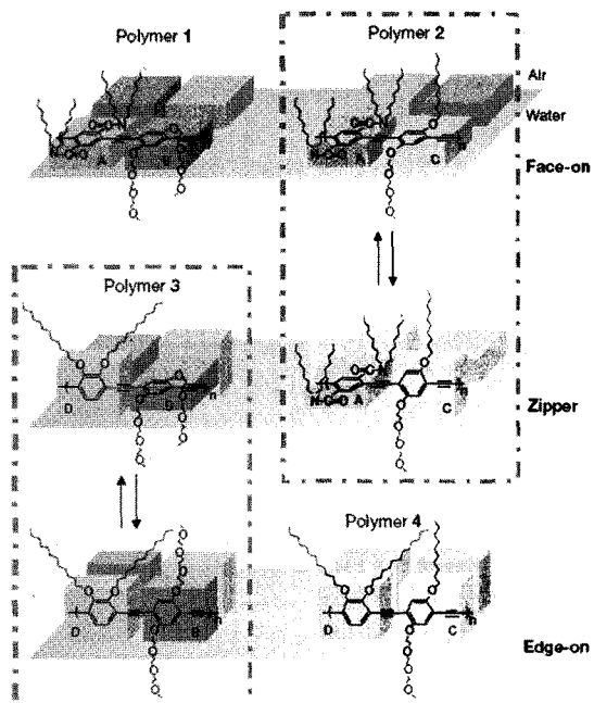
그림 1. 형광 공역 고분자의 conformation 변화에 따른 발광파장의 변화. 뒤틀림 구조에 의한 공역 길이 저하에 따른 발광파장의 단파장 이동과 평면화에 기인한 공역길이 증대에 따른 발광파장의 장파장 이동현상 발생. 3
