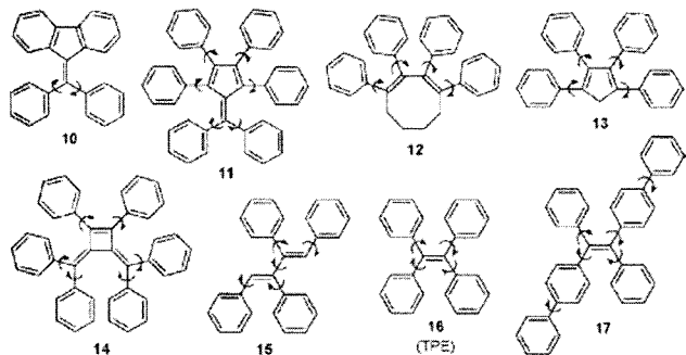
그림 14. 오직 순수한 탄화수소만으로 이루어져있는 AIE 형광체들의 예.
