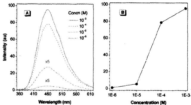
그림 9. 이치환형 아세틸렌폴리머의 형광방출 스펙트럼 (A) 농도에 따라 강도만 증가하고 파장은 변하지 않는 형광방출 스펙트럼 (B) 농도에 따른 형광강도 플롯.
