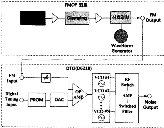
그림 12. FMOP 제어회로를 이용한 잡음신호발생
