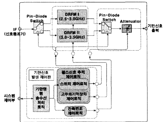
그림 5. 기만신호발생기 구성도
