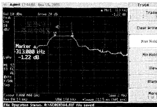
그림 23. 속도기만(RGPO+VGPI) 주파수특성
