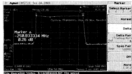
그림 33. 점소인 대역폭(256MHz)
