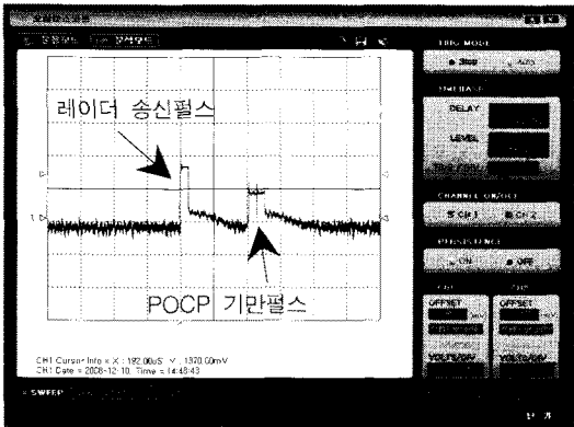
그림 35. POCP 기만신호의 펄스특성
