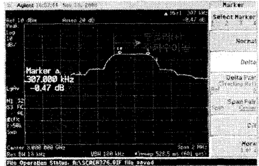
그림 25. 속도기만(RGPI+VGPO) 주파수특성
