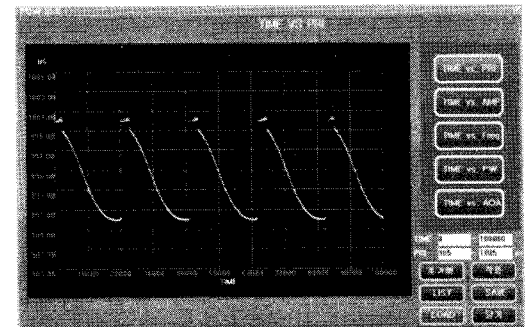
그림 21. 거리기만(RGPI)-시간대 펄스반복주기 특성
