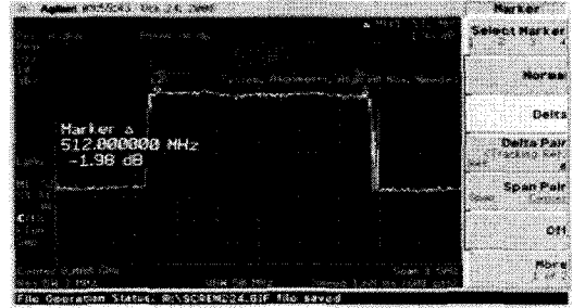
그림 31. 광대역 잡음(512MHz)
