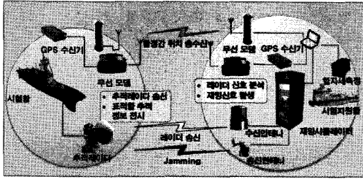
그림 34. 해상시험 구성도
