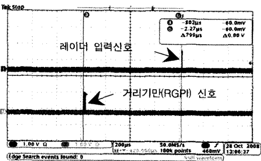
그림 24. 속도기만(RGPI+VGPO) 펄스특성
