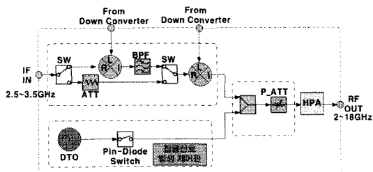
그림 11. 주파수 상향변환 및 잡음재밍
