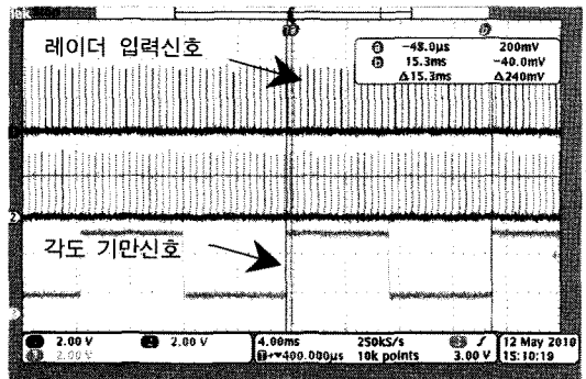
그림 26. 각도기만 시간특성
