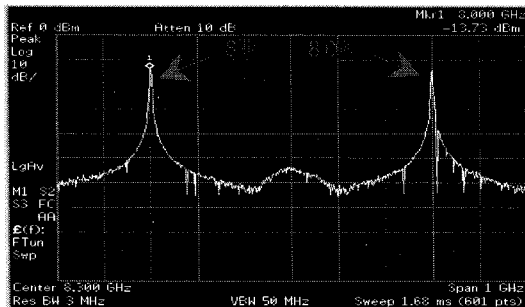
그림 17. 레이더 모사신호
