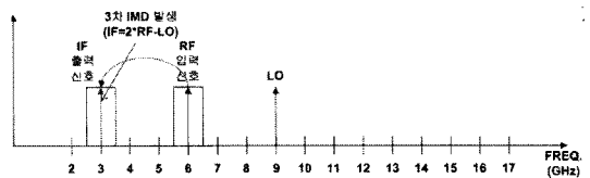
그림 2. 1차 하향변환에 의한 IF 밴드폭내 상호변조신호 발생
