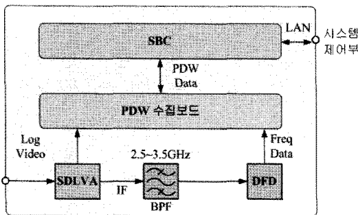
그림 4. 신호처리기 구성도
