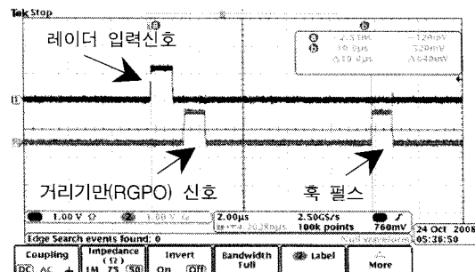
그림 18. 거리기만(RGPO) 펄스특성
