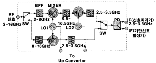
그림 1. 주파수 하향변환 구성도
