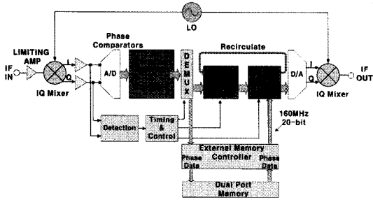
그림 6. DRFM 처리 구성도
