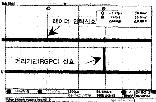
그림 22. 속도기만(RGPO+VGPI) 펄스특성
