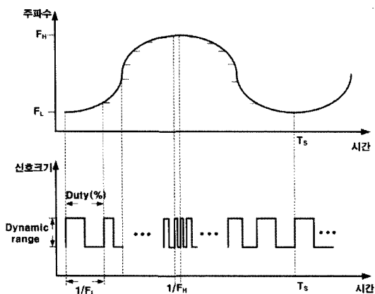
그림 10. 각도기만(비선형 소인) 구현 방식
