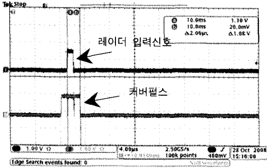
그림 28. 커버펄스 시간특성
