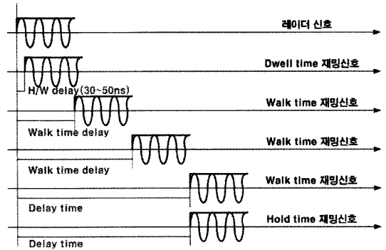
그림 8. 거리기만 개념
