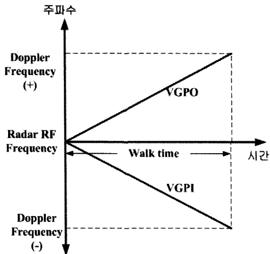
그림 9. 속도기만 구현 방식
