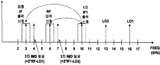
그림 3. 1, 2차 하향변환에 의한 IF 밴드폭내 상호변조신호 제거
