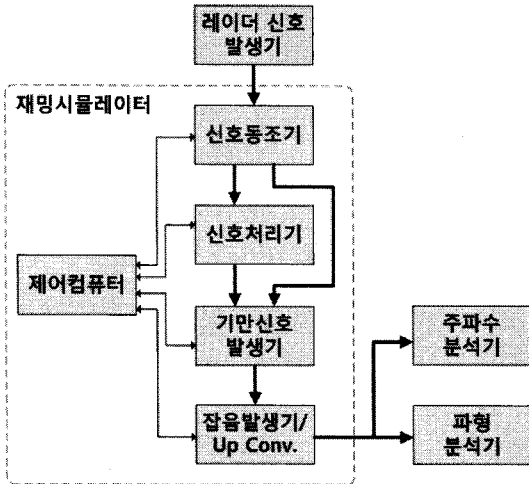
그림 16. 실험장비 구성도
