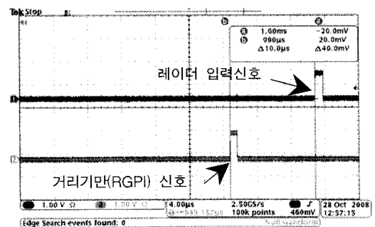
그림 20. 거리기만(RGPI) 펄스특성
