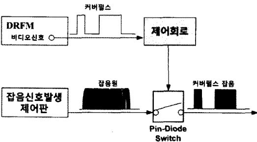
그림 13. 커버펄스 잡음
