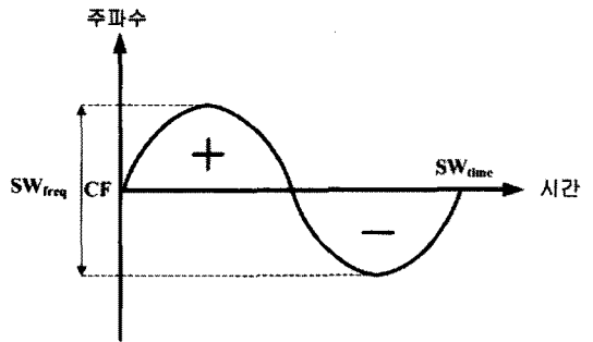
그림 15. 점소인 형태(정현파)
