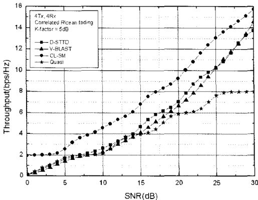
그림 5. 라시안 환경에서 (4×4) MIMO 시스템의 스펙트럼 효율 비교
