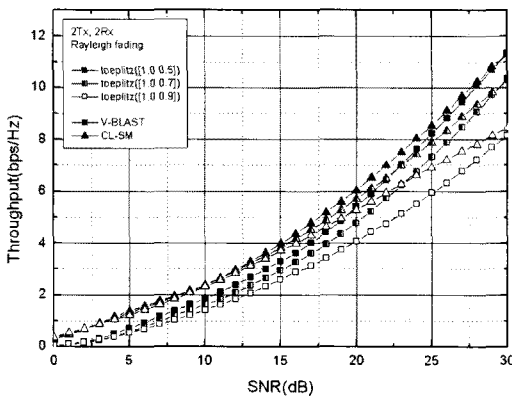
그림 2. 코릴레이션이 (2×2) 공간 다중화 기법의 스펙트럼 효율에 미치는 영향
