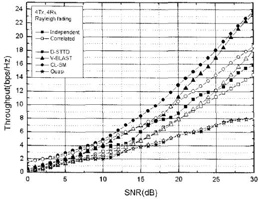
그림 4. 레일리 환경에서 (4×4) MIMO 시스템의 스펙트럼 효율 비교
