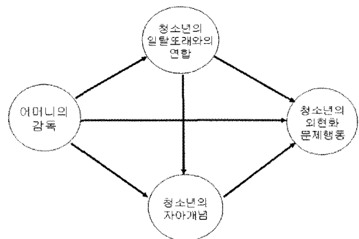
<그림 1> 연구모형
