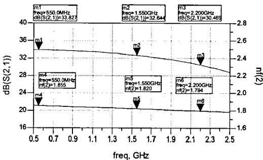
그림 8. 광대역 2단 저잡음 증폭기 모의실험 결과
