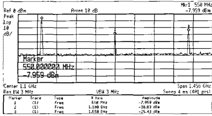
a) 550 MHz 발진기 출력 스펙트럼
