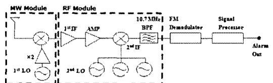
그림 1. 레이더 탐지기의 전체 시스템 개략도
