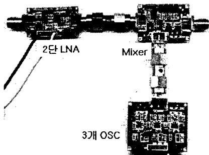
그림 13. RF 모듈단 제작된 실물 사진
