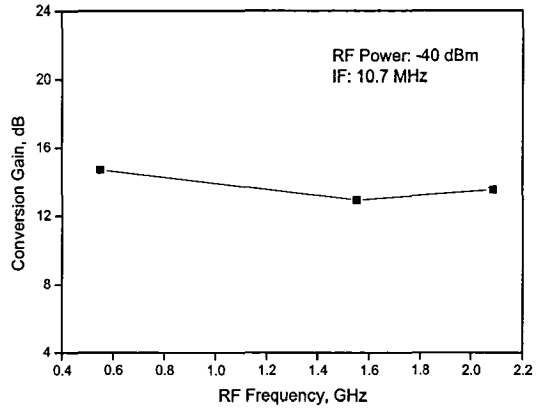
그림 15. 혼합기의 변환 이득 측정 결과
