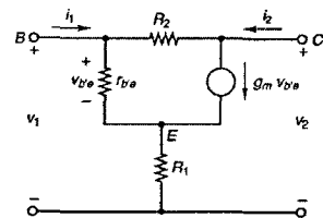
그림 3. BJT 소자의 부캐환 회로에 대한 소신호 등가회로
