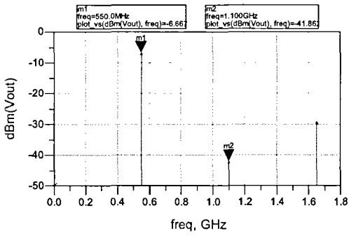
a) 550 MHz 발진기 출력 스펙트럼
