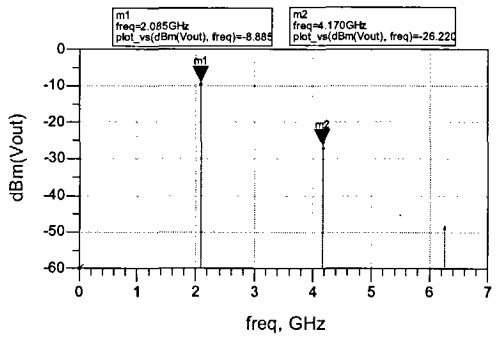
c) 2085 MHz 발진기 출력 스펙트럼
