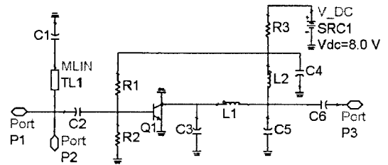
그림 9. 혼합기 회로도
