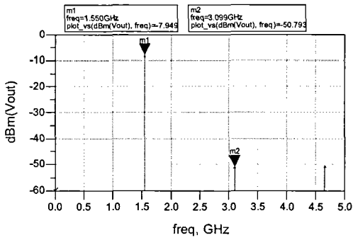
b) 1550 MHz 발진기 출력 스펙트럼
