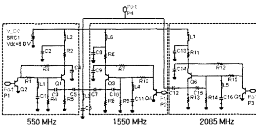
그림 11. 3개 발진기 회로도
