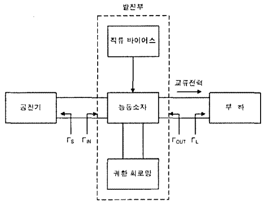
그림 6. 발진기의 기본 블록도
