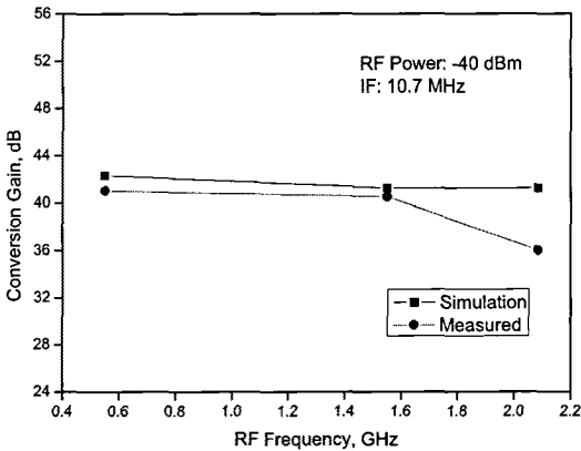
그림 17. RF 모듈단의 변환 이득 모의실험 및 측정 결과
