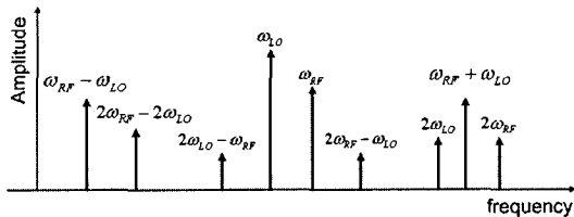
그림 5. 혼합기의 출력 스펙트럼
