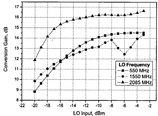
그림 10. 혼합기 변환 이득 모의실험 결과
