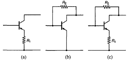
그림 2. 부캐환 회로의 구조
