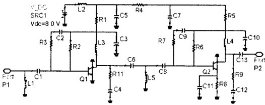
그림 7. 광대역 2단 저잡음 증폭기 회로도
