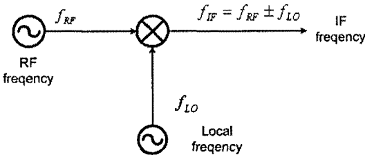
그림 4. 주파수 혼합기의 하향 변환 구조도
