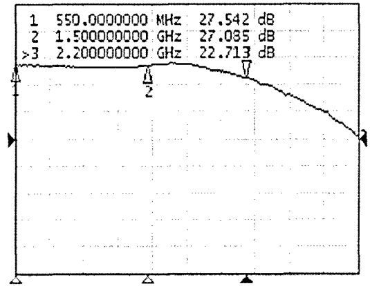
그림 14. 광대역 2단 저잡음 증폭기 측정 결과
