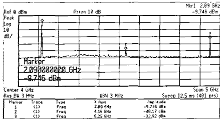
c) 2085 MHz 발진기 출력 스펙트럼
