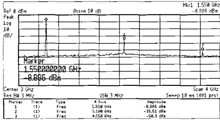
b) 1550 MHz 발진기 출력 스펙트럼
