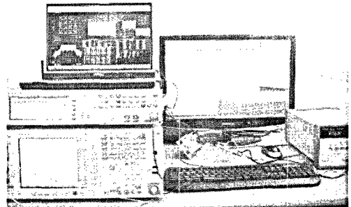
그림 5. RF 송·수신기 IC의 테스트 환경
