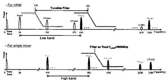
그림 3. 송신부의 고조파 성분 억압특성
