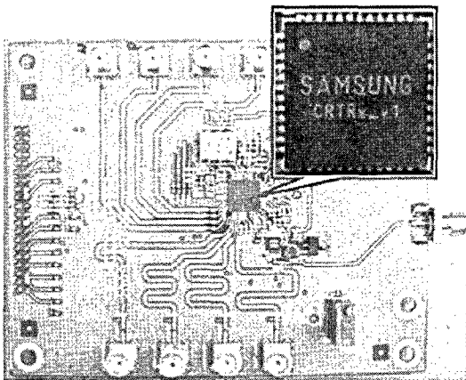
그림 4. 제작된 CMOS RF 송·수신기 IC의 테스트 보드
