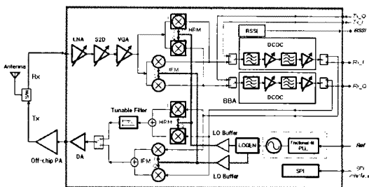
그림 2. 개발된 CMOS RF 송·수신기 IC의 구조
