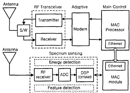
그림 1. WRAN 시스템 단말의 Block diagram
