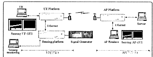
그림 10. 개발된 인지무선 기술 기반의 WRAN 시스템 연동 구성도
