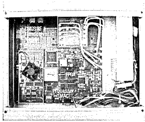
그림 9. 개발된 WRAN 시스템 플랫폼 내부사진
