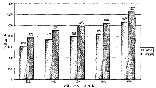
그림 5. 소멸되는 노드 비율에 따른 라운드 수 비교 Fig. 5. Energy consumption rate of node disappearance
