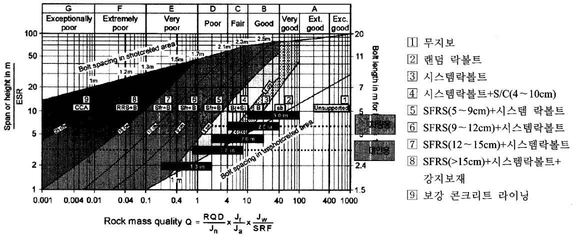
그림 1. Q-system 도표를 이용한 지보량 선정(Barton & Grimstad, 1994)
