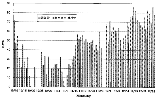
[그림 10] 태양열 집열량 및 지열히트펌프 생산열량
