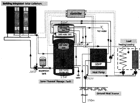
[그림 7] 태양열+지열 하이브리드시스템 개요도
