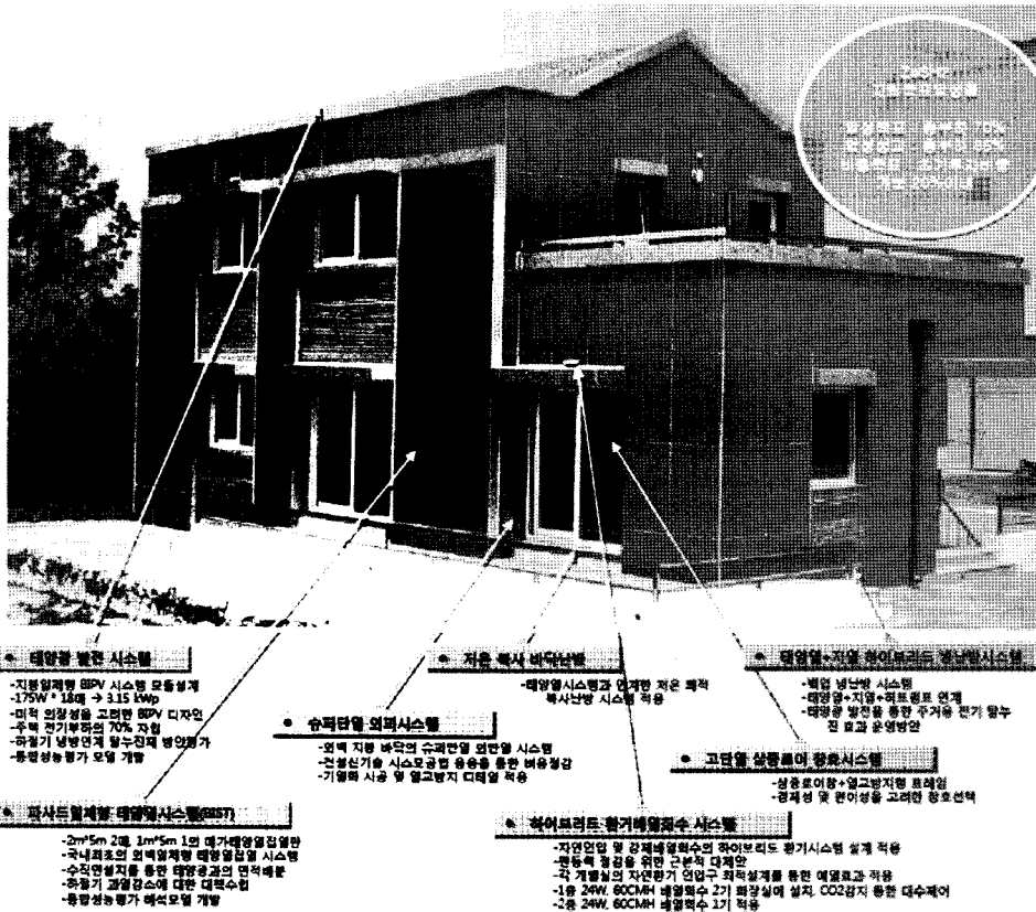
[그림 6] ZeSH-II에 적용된 핵심기술
