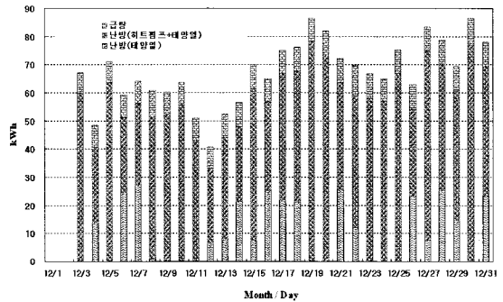
[그림 11] 축열조 및 향온조에 의한 난방 및 급탕공급량
