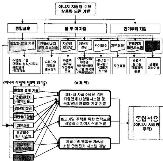
[그림 2] 건물에너지 자립화를 위한 요소기술의 통합
