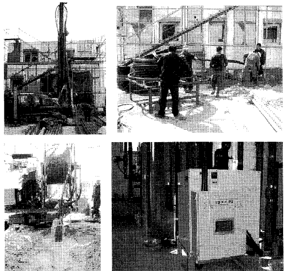
[그림 8] 태양열+지열 하이브리드시스템 설치시공 사진
