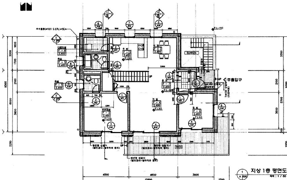
[그림 3] ZeSH-II 1층 평면도
