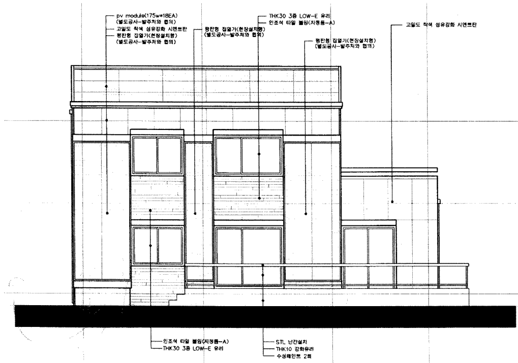
[그림 4] ZeSH-II 남측면도
