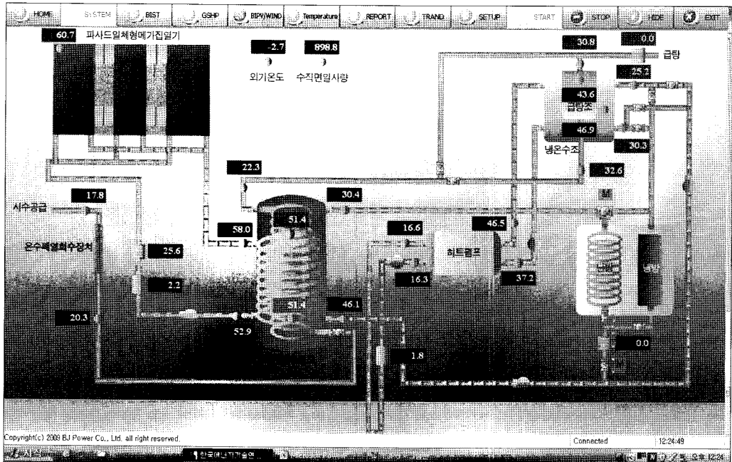
[그림 9] 태양열 + 지열이용 히트펌프시스템 모니터링 화면
