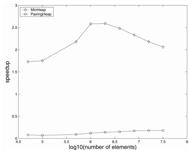
(그림 4) 무작위 모델에서의 성능 : 실행 시간(왼쪽) 및 상대성능(오른쪽)
