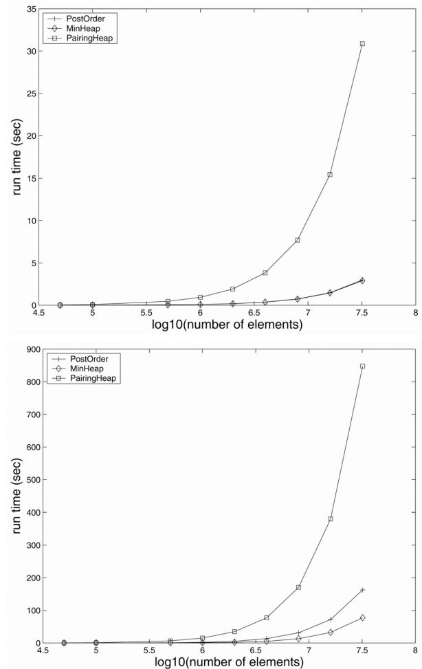
(그림 2) 기본 모델에서의 실행 시간 : 삽입(위) 및 삭제(아래)
