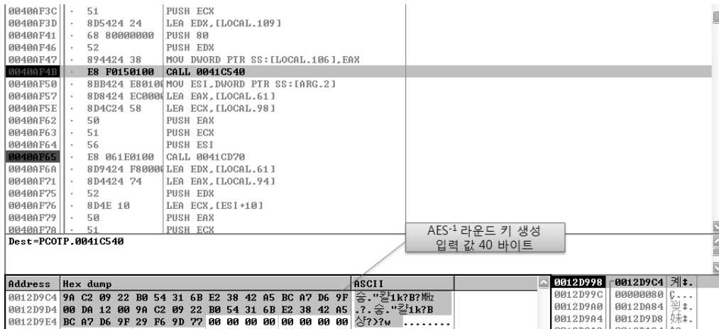
(그림 12) AES 복호화 라운드 키 생성 40 바이트 입력값
