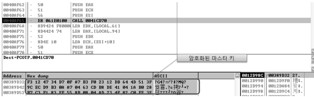
(그림 13) 암호화된 마스터 키 정보
