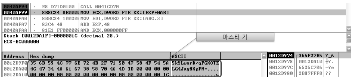
(그림 15) 복호화된 마스터 키
