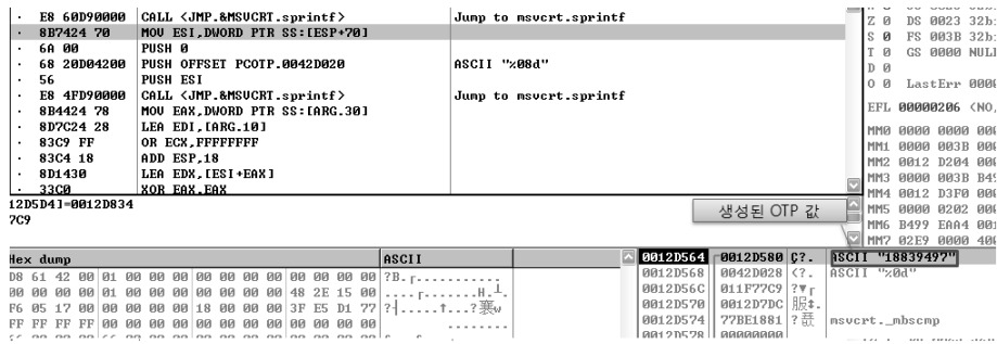
(그림 19) 역공학을 통해 확인한 OTP 값
