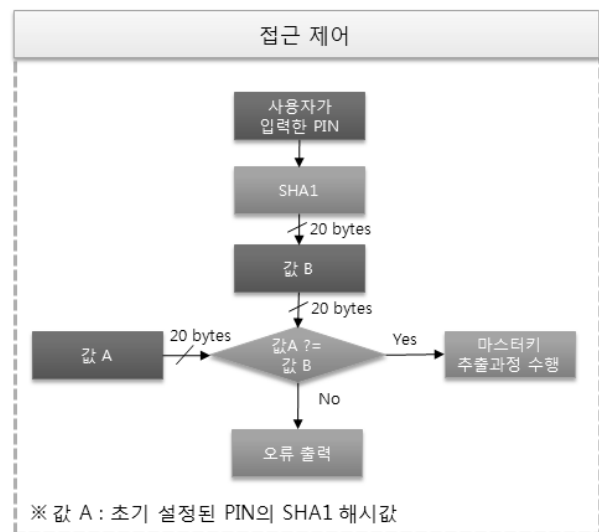
(그림 6) 접근제어
