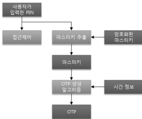
(그림 5) PC에 탑재된 OTP의 동작 과정
