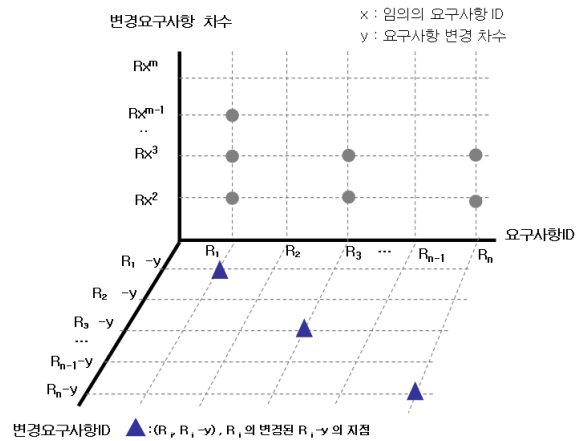
(그림 7) 추적테이블에서 변경율 산정
