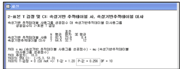
(그림 12) 2-표본 t 검정 결과
