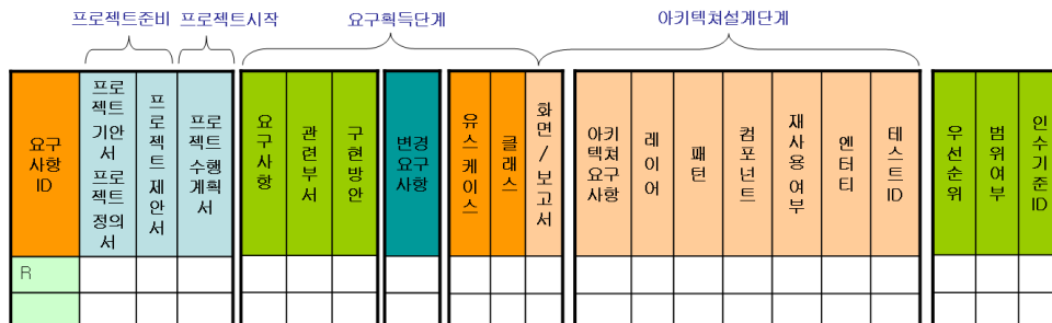
(그림 1) 기능요구사항추적테이블
