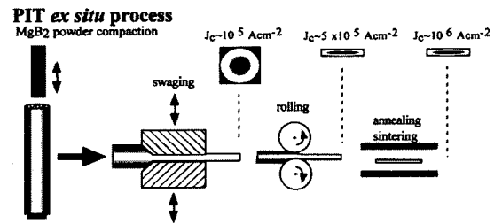
그림 2. MgB 2 초전도 선재제조 공정도 (ex situ).
