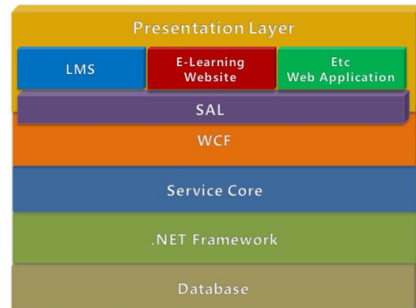
그림 2. SOA 기반의 LMS 모델
