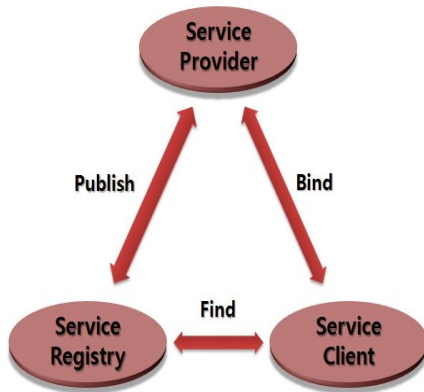
그림 1. SOA 구성 요소간의 상호 관계
