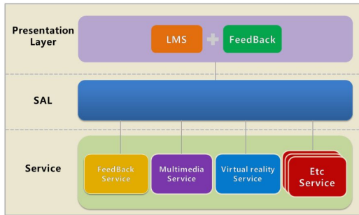
그림 3. SAL을 통한 어플리케이션의 기능 추가
