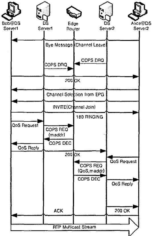
그림 9. 채널 변경 과정
