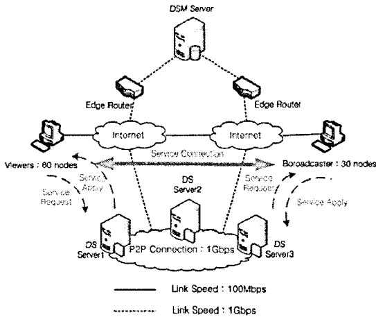
그림 10. 시뮬레이션 네트워크 모델
