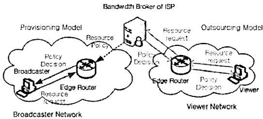
그림 6. COPS의 동작 과정
