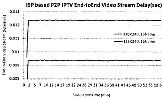
그림 12. P2P 기반 IPTV에서 비디오 전송 지연시간
