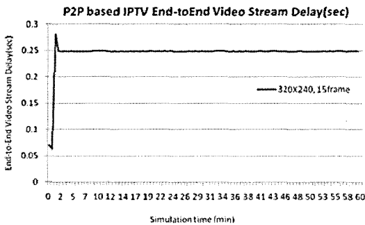
그림 13. ISP 기반 P2P IPTV의 비디오 전송 지연시간
