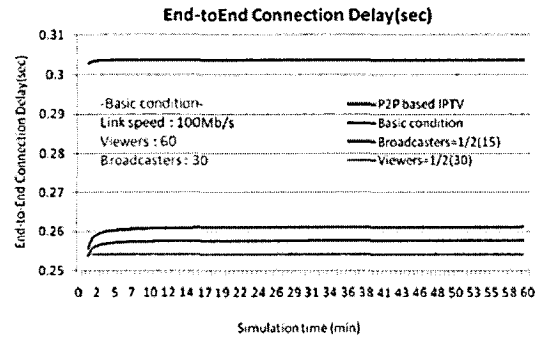
그림 11. ISP 기반 P2P IPTV의 연결 지연시간
