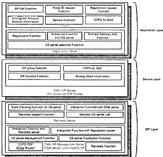
그림 3. ISP 기반 P2P IPTV의 기능적 계층구조
