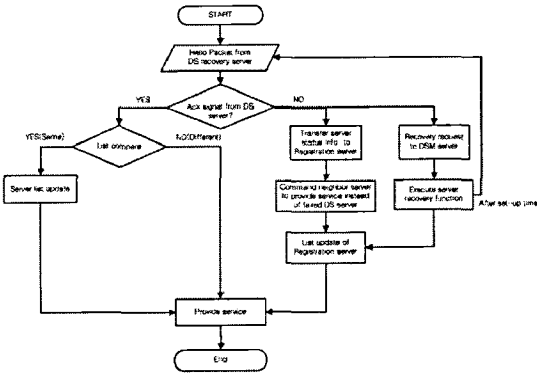
그림 4. DNS-SIP 서버 복구 메커니즘의 흐름도
