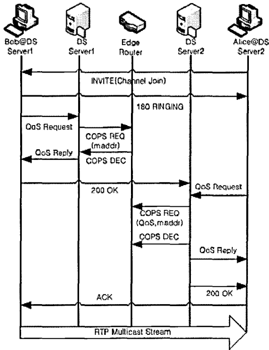
그림 8. 기존 사용자간의 세션 연결
