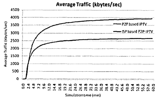
그림 14. 네트워크에 존재하는 평균 트래픽량 비교
