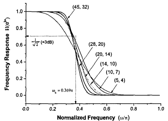
그림 2. (N, K) 에 따른 H_0(e^{jw}) 응답 특성
