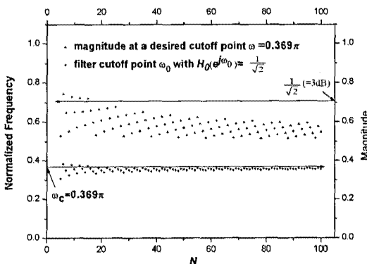
그림 1. 식(18)에 의한 H_0(e^{jw}) 의 실제 차단주파수 응답특성
