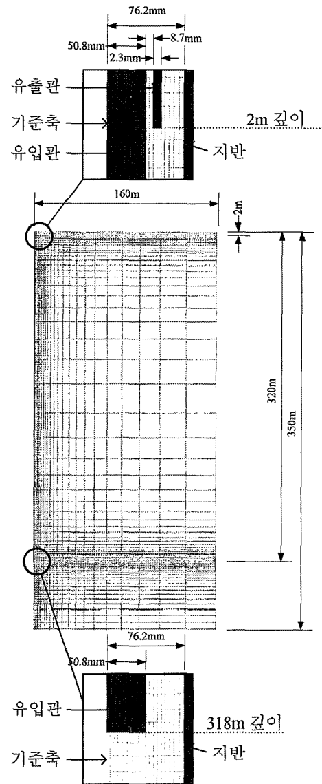
그림 6. Mikler(1993) 자료검증에 사용된 해석영역과 요소망
