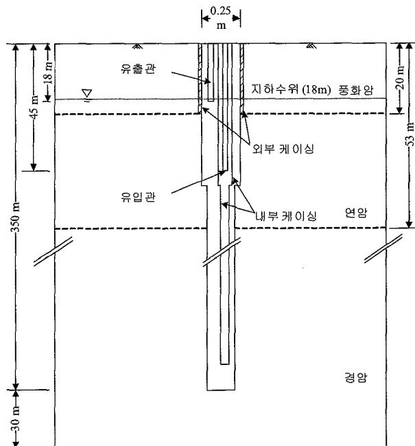
그림 9. 의령 체육진흥센터 SCW 개략도
