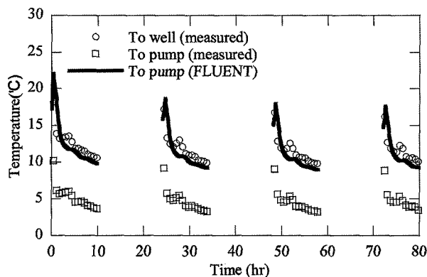
그림 12. 80시간 가동주기 동안의 의령군 현장 계측 데이터와 수치해석결과 비교
