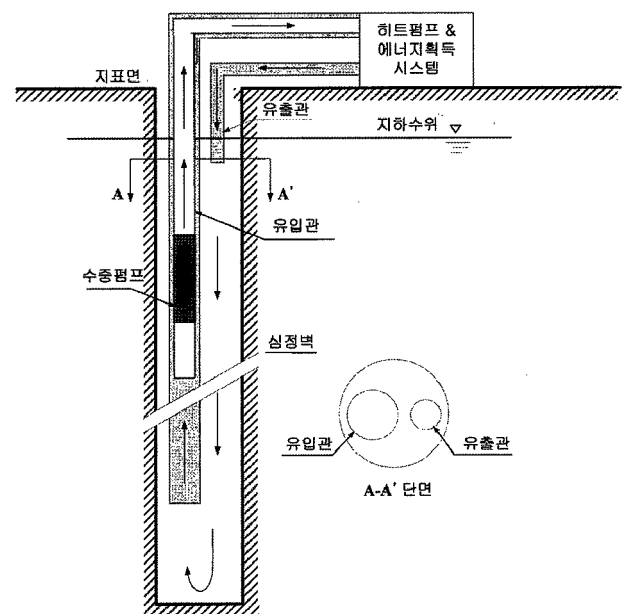
그림 1. 단일심정시스템의 개략도
