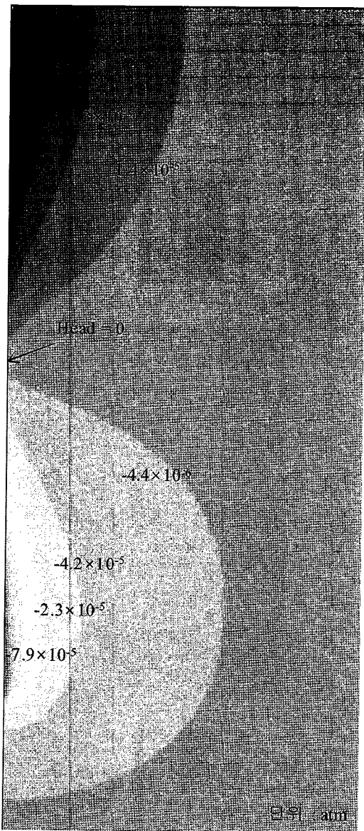
그림 7. 지반에서 계산된 압력수두 분포
