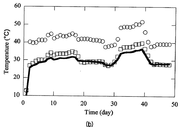
그림 8. Pennsylvania SCW에서 측정된 유입수(Mikler, 1993) 및 계산된 유입수 온도 비교
