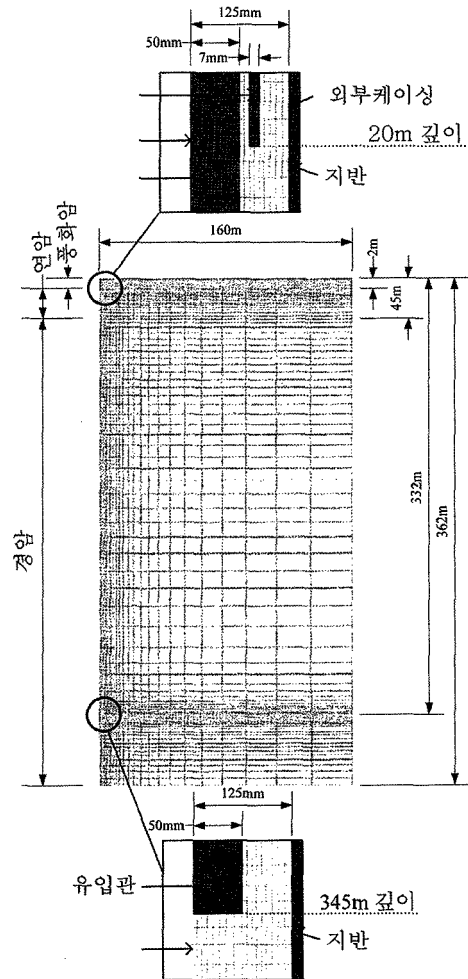
그림 10. 의령 체육진흥센터 자료 검증에 적용된 해석영역과 요소망
