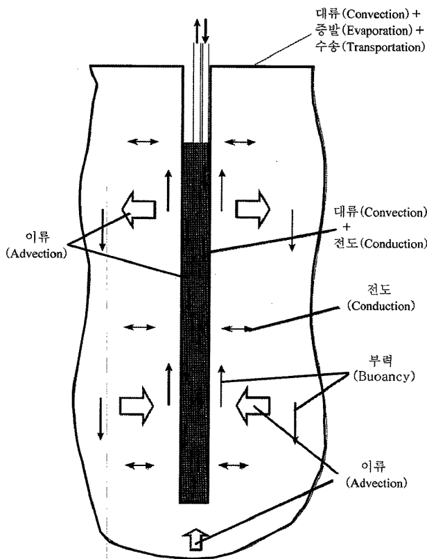
그림 2. SCW 시스템의 열 이동 메커니즘(Rees 등, 2004)
