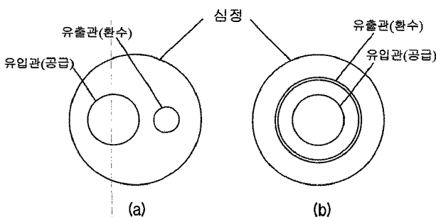
그림 3. SCW 단면 (a) 실제형상, (b) 축대칭해석에서 적용된 등가환산 형상
