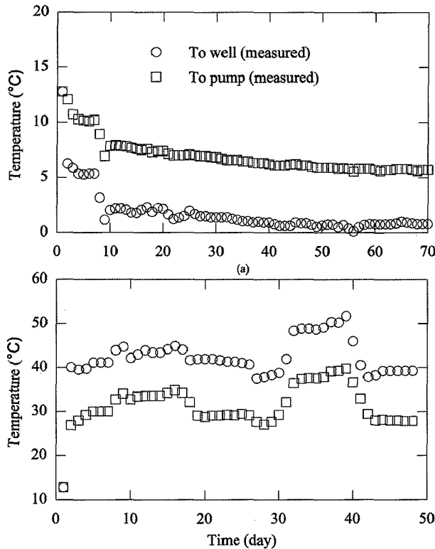
그림 5. Pennsylvania에 설치된 SCW에서 측정된 유출수 및 유입수 온도(Mikler, 1993)
