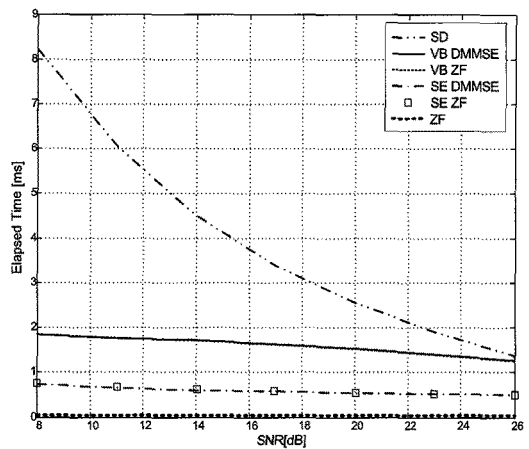
그림 8. 2x2 MIMO 시스템에서 각 알고리즘의 수행시간
