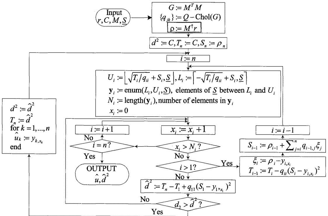
그림 2. VB SD 알고리즘 [5]
