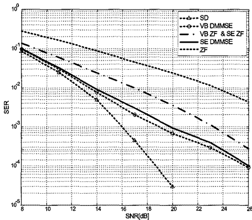
그림 7. 2x2 MIMO 시스템에서 SER 성능비교
