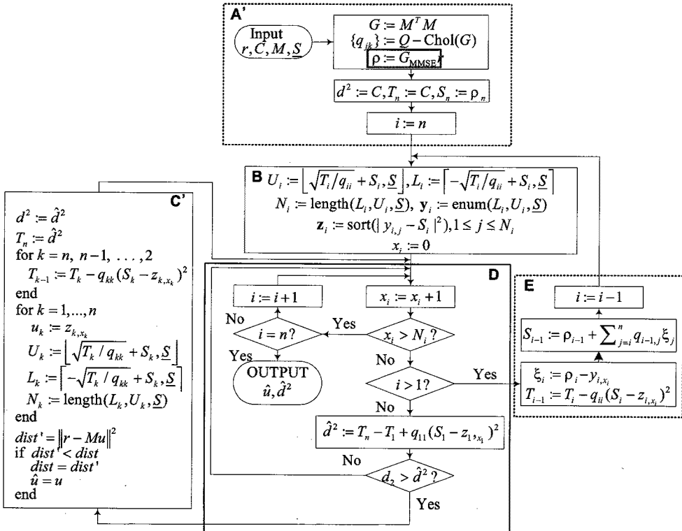
그림 6. 제안 알고리즘
