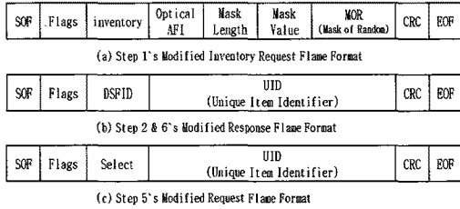
그림 12. 제안한 프로토콜의 수정된 프레임 포맷
