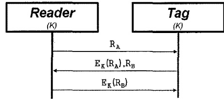
그림 2. Challenge-Response Protocol
