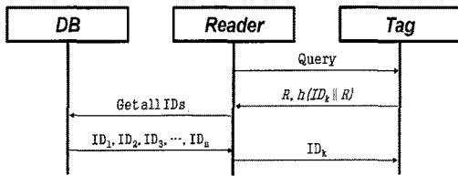
그림 1. Randomized-Hash Lock Protocol
