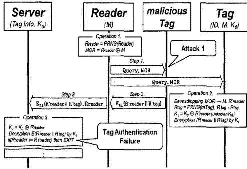
그림 13. 위장 태그를 통한 공격 시나리오 1
