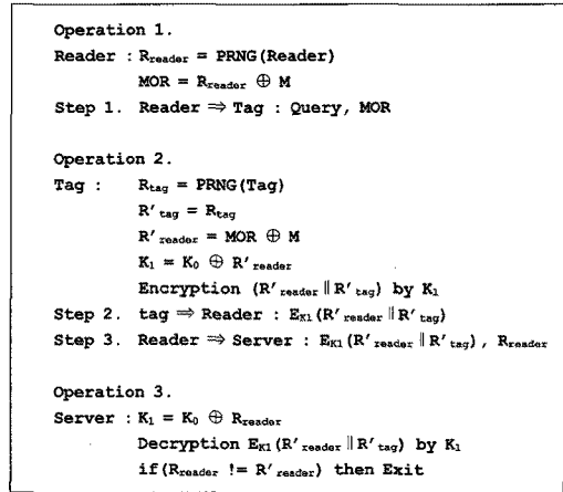
그림 7. 태그 인증 동작 코드
