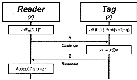
그림 3. HB Protocol
