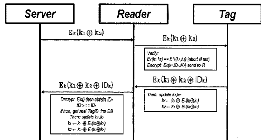
그림 4. B. Toirul의 Mutual-Authentication Protocol
