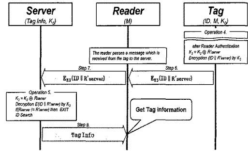
그림 10. 태그의 정보 획득 과정
