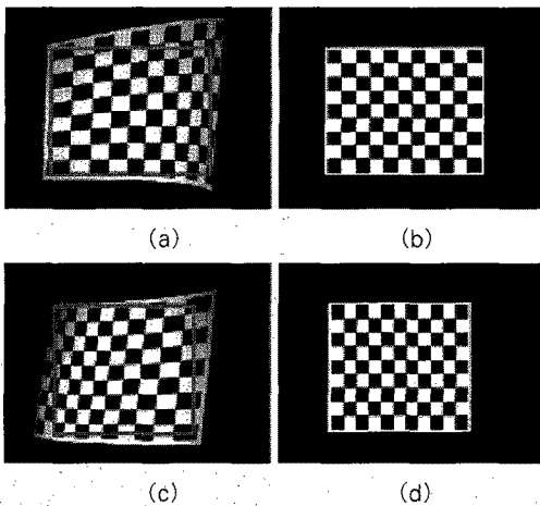
그림 6. (a)오목한 스크린에 영상을 투여한 후 카메라로 촬영한 영상, (b)(a)의 보정영상, (c) 불룩한 형태의 스크린에 영상을 투여한 후 카메라로 촬영한 영상, (d) (c)의 보정영상
