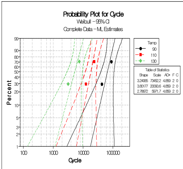
그림 6 3가지 스트레스 수준의 와이블 선도
