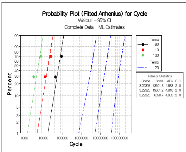
그림 7 와이블-아레니우스 선도
