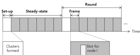
(그림 1) LEACH의 Time Line
