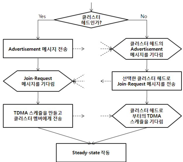
(그림 2) LEACH의 동작 절차
