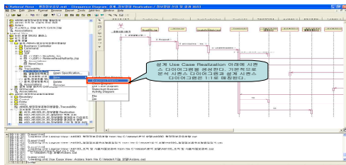
그림 6. 설계 컴포넌트 상호작용 다이어그램 생성 Fig. 6. Formation of Design Component Interaction Diagram
