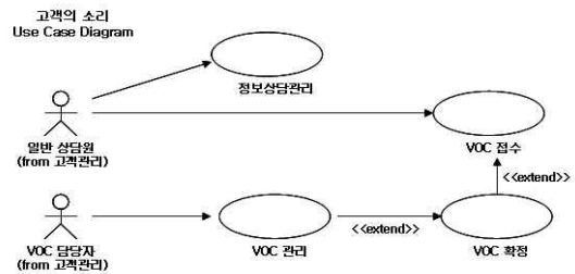
그림 2. Use Case 다이어그램 Fig. 2. Use Case Diagram
