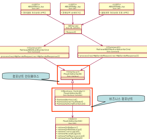
그림 7. 설계 컴포넌트 구조 모델링 Fig. 7. Modeling of Design Component Structure
