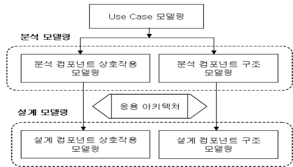
그림 1. 모델링 진행 절차 Fig. 1. Procedure of Modeling Progress
