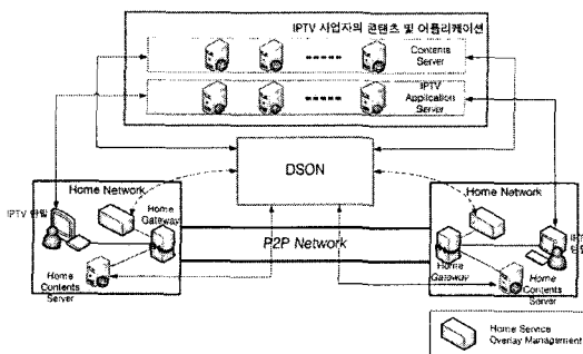
그림 10. DSON 기반의 홈 네트워크 기능 구조
