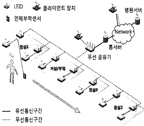
그림 1. 유헬스 시스템 구성도 Fig. 1. u-Health System Organization
