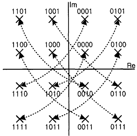
그림 1. APSLM에서 Gray 사상을 이용한 16-QAM 성상도의 예시
