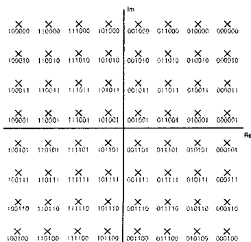
그림 2. Gray 사상을 사용한 64-QAM 성상도의 예시
