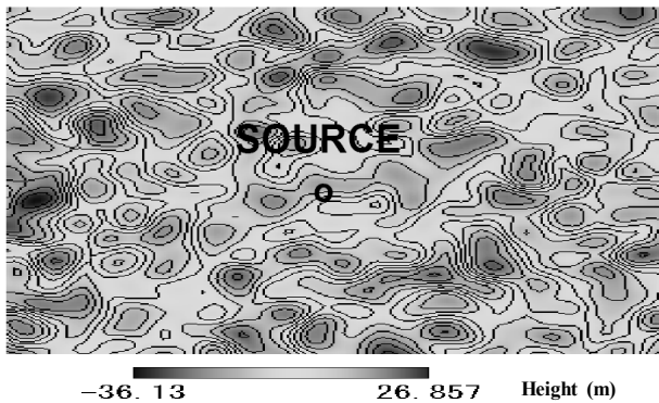
그림 2 2차원 불규칙 조면의 구조와 파원 Fig. 2 Geometry of 2D rough surface and source.
