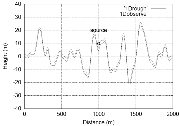
그림 1 1차원 불규칙 조면의 구조와 파원 Fig. 1 Geometry of 1D rough surface and source.
