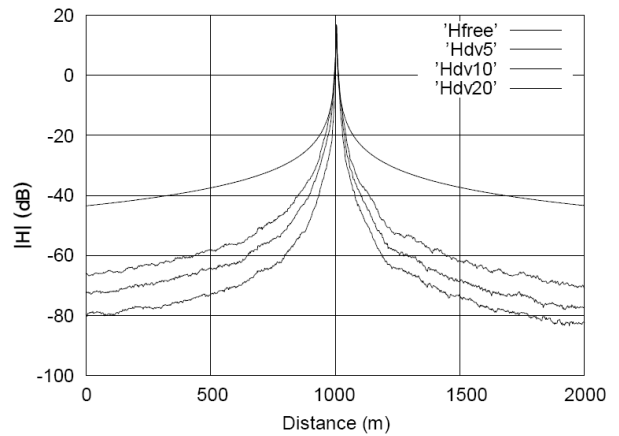
그림 8 dv 의 변화에 의한 전계분포(H-wave) Fig. 8 H-wave distributions with dv as a parameter.
