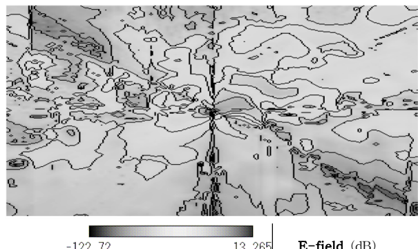
그림 14 전계분포(수평편파에 대한 second order ray) Fig. 14 Field computed by second order rays for horizontal polarization ( c=50 m, dv=5 m, sl=1 Km).
