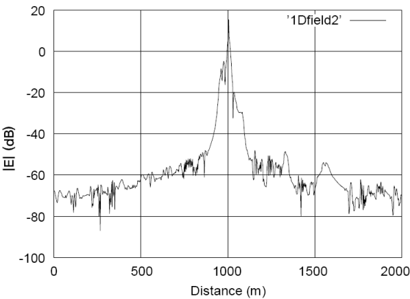
그림 5 전계강도(second order ray) Fig. 5 Field computed by second order ray.
