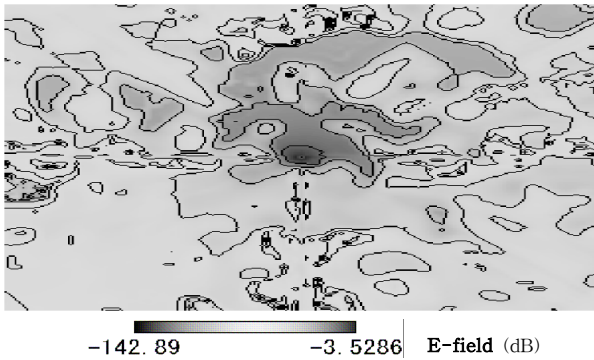
그림 11 전계분포(수직편파에 대한 first order ray) Fig. 11 Field computed by first order rays for vertical polarization ( c=50 m, dv=5 m, sl=1 Km).
