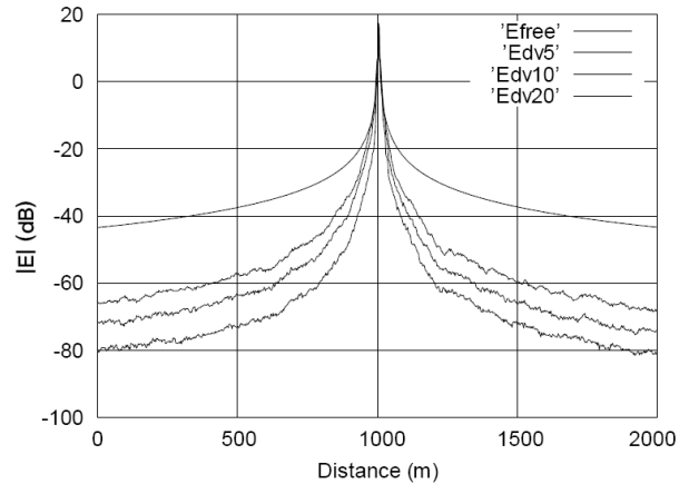
그림 7 dv 의 변화에 의한 전계분포(E-wave) Fig. 7 E-wave distributions with dv as a parameter.
