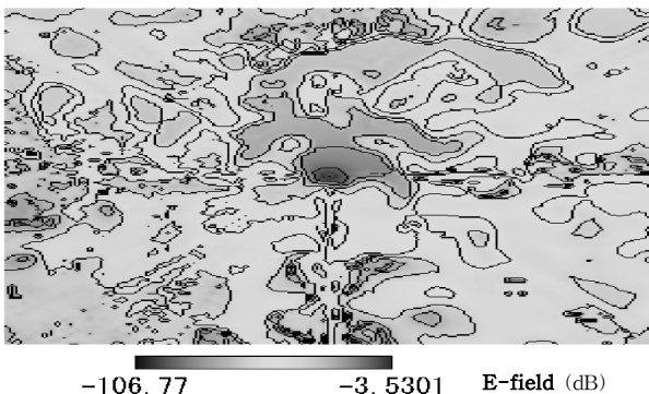
그림 13 전계분포(수직편파에 대한 second order ray) Fig. 13 Field computed by second order rays for vertical polarization ( c=50 m, dv=5 m, sl=1 Km).
