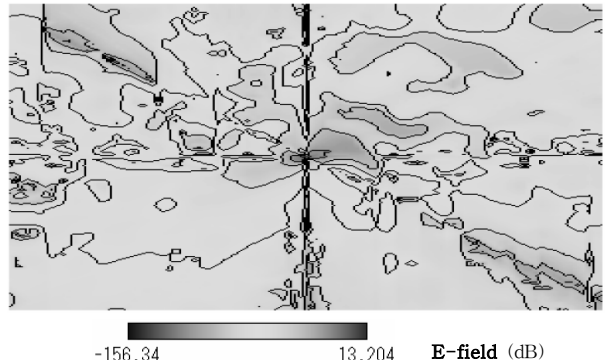
그림 12 전계분포(수평편파에 대한 first order ray) Fig. 12 Field computed by first order rays for horizontal polarization ( c=50 m, dv=5 m, sl=1 Km).
