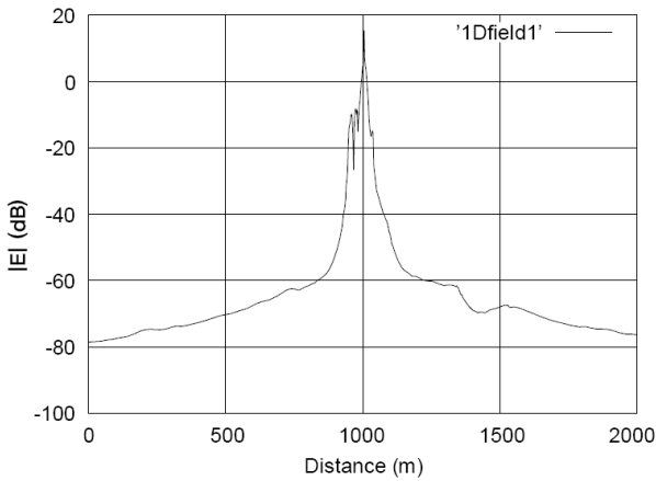
그림 4 전계강도(first order ray) Fig. 4 Field computed by first order ray.
