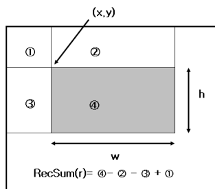
그림 2. 픽셀 합 Fig. 2 The Total Number of Pixels
