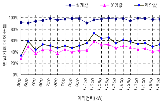
그림 5. 단위세대 부하용량 조정에 따른 변압기 최대이용률의 비교
