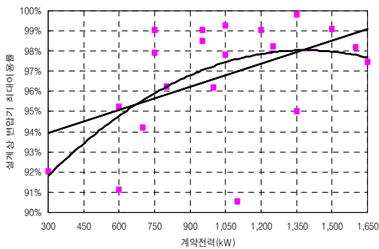
그림 3. 변압기최대이용률의 설계값 산점도와 회귀모형 Fig. 3. Scatter plot of the value of design of a maximum utilization factor and linear regression model
