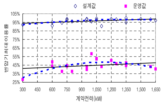
그림 4. 변압기최대이용률의 설계값과 운영값의 산점도와 회귀모형
