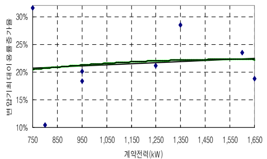
그림 2. 조사고객의 5년간 변압기최대이용률의 증가율 산점도와 회귀모형
