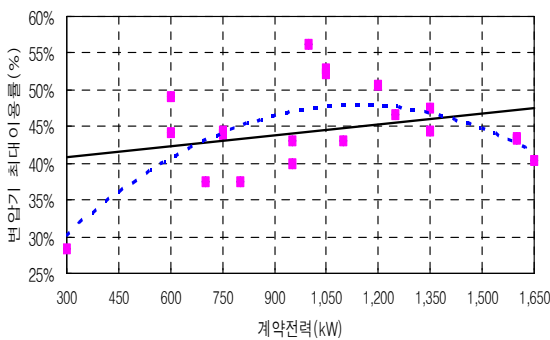
그림 1. 변압기최대이용률 산점도와 회귀모형 Fig. 1. Scatter plot of maximum utilization factor of transformer and linear regression model
