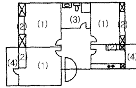
<그림 1>1970년대 말 층집 예(66㎡)
