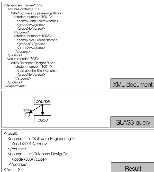
(그림 6) GLASS 질의 처리의 예
