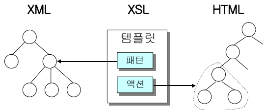
(그림 2) XSL의 패턴과 템플릿
