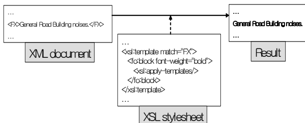
(그림 3) XSL 질의 처리 예
