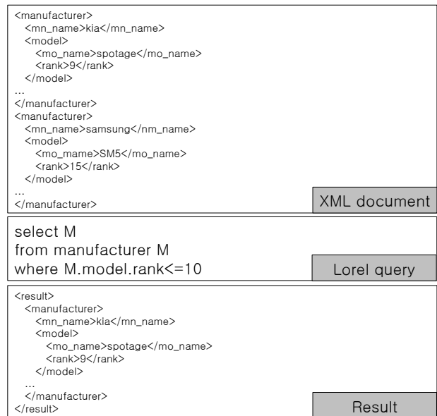
(그림 7) Lorel 질의 처리의 예
