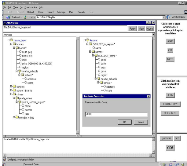
(그림 5) BBQ 실행 화면의 예
