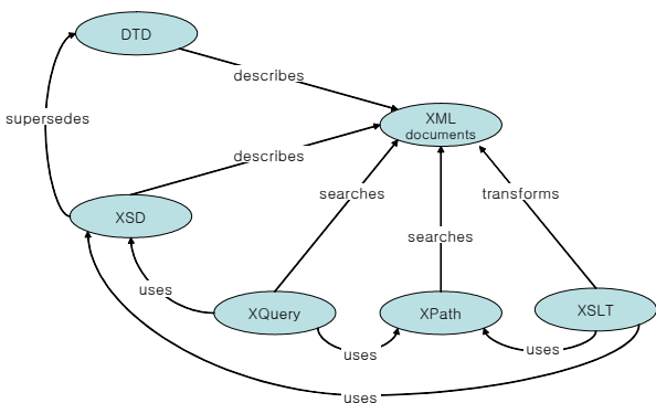
(그림 12) XML 명세화 도구간의 관계성
