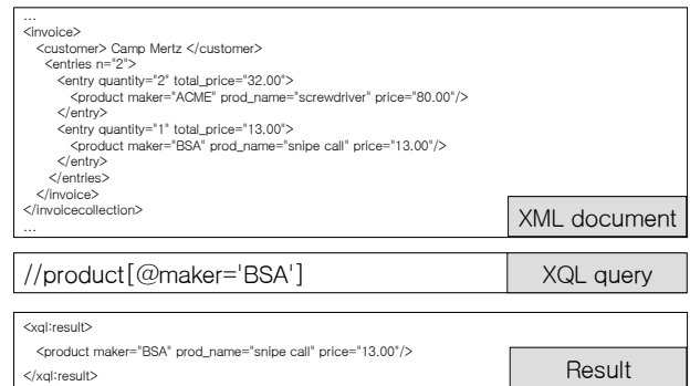
(그림 4) XQL 질의 처리의 예
