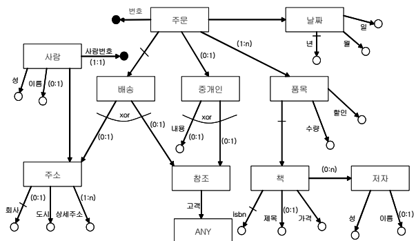
(그림 27) XML-GDM으로 표현한 "주문.dtd"
