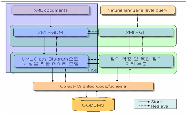
(그림 25) UML 클래스 다이어그램으로 사상을 위한 데이터 모델
