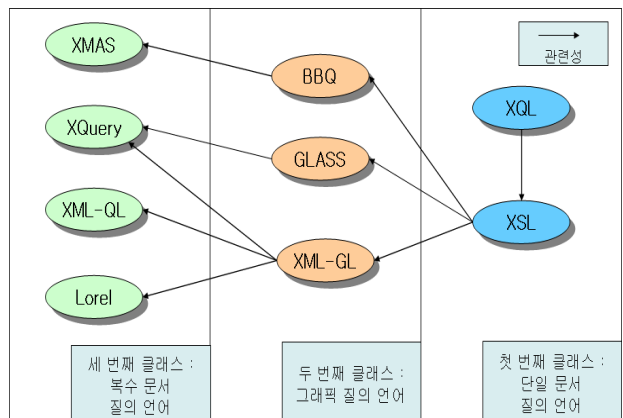
(그림 1) XML 질의 언어의 클래스별 분류
