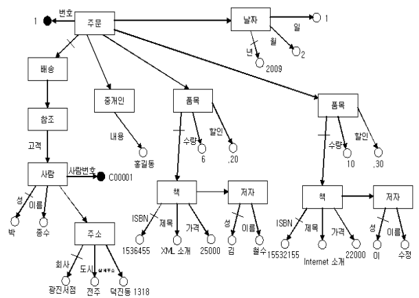
(그림 30) 도서관련 XML 문서를 XML-GL로 표현
