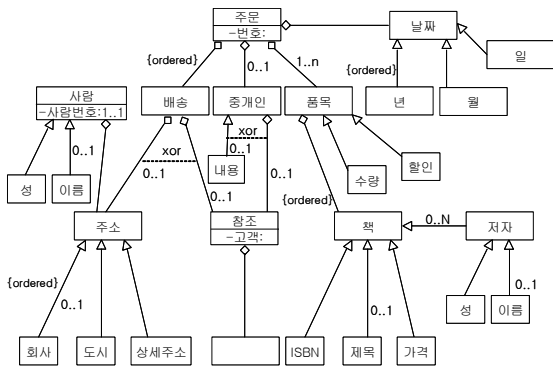
(그림 28) UML 클래스 다이어그램으로 표현한 "주문.dtd"
