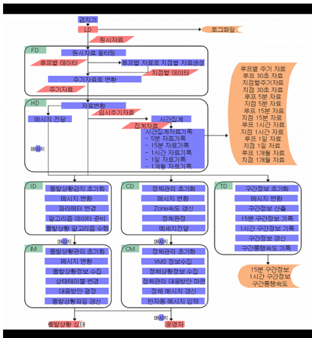
(그림 1) FTMS 자료 처리 흐름도
