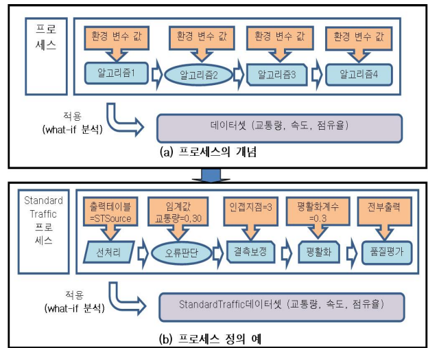
(그림 4) 교통이력 데이터의 what-if 분석을 위한 프로세스 개념과 프로세스 정의 예
