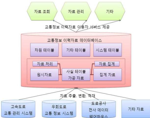
(그림 2) 통합 교통이력 데이터베이스 시스템의 구조
