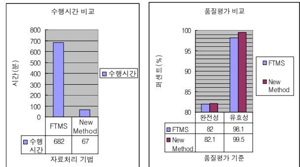
(그림 15) 기존의 FTMS 기법과 제안한 기법의 자료처리 성능 비교
