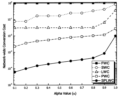
그림 6. \alpha 값에 따른 네트워크 파장 변환 비용
