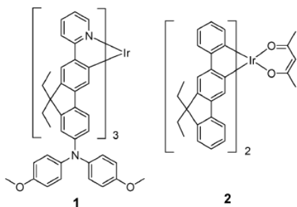
그림 3. 황색 인광 dopant의 구조.
