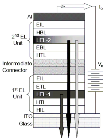
그림 1. 고효율/장수명 백색 tandem 구조 소자.
