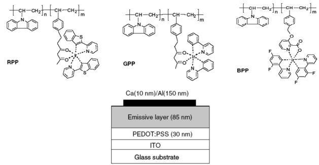
그림 8. 대표적인 청색형 청색, 녹색, 적색의 고분자 구조와 소자 구조.
