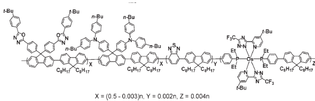
그림 7. Osmium complex를 도입한 백색 발광 고분자 구조.
