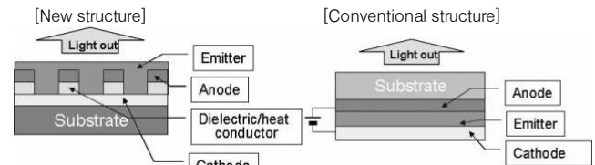
그림 9. Showa-Denko의 신규 소자 구조와 백색 면광원.
