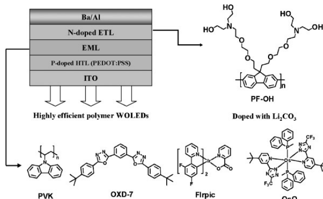
그림 4. 전자 수송 고분자를 이용한 적층형 소자 구조와 화합물 구조.
