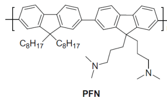
그림 4. 전자 수송 고분자를 이용한 적층형 소자 구조와 화합물 구조.
