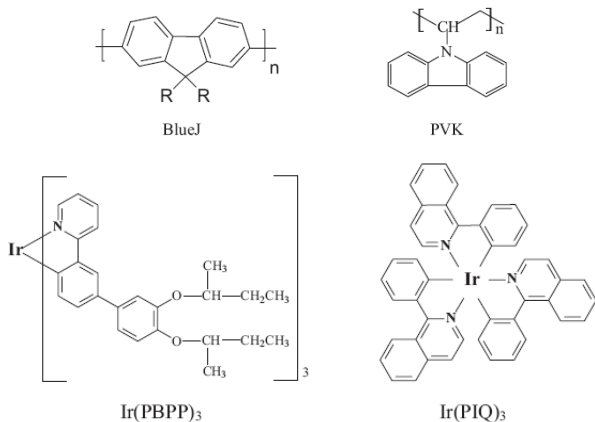
그림 2. 청색 고분자, 녹색 인광, 적색 인광과 host PVK의 화합물 구조.
