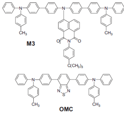
그림 6. 단일계 백색 고분자에 적용한 적색 단량체 구조.
