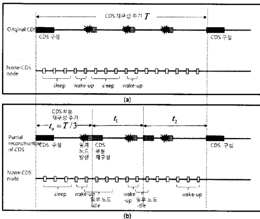
그림 8. CDS 재구성 주기 예: (a)기존 방식, (b) 부분 재구성 방식
