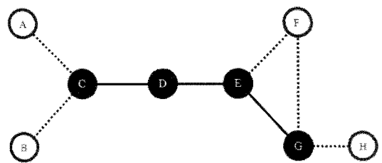
그림 1. 연결형 dominating set 예
