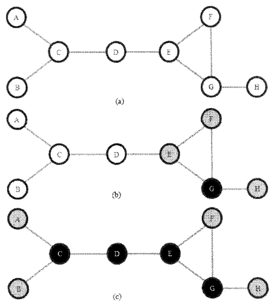
그림 3. Guha와 Kuller 알고리즘 적용 예
