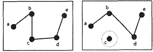
(a) CDS 기반 토폴로지 구성 (b) 임계 노드가 c 일 때
