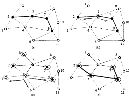
그림 7. CDS 부분 재구성 예
