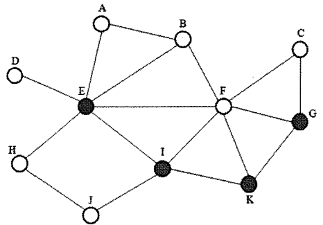
그림 6. 트래픽 망을 고려한 CDS 구성
