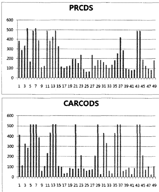
그림 14. 각 노드의 배터리 잔량 비교
