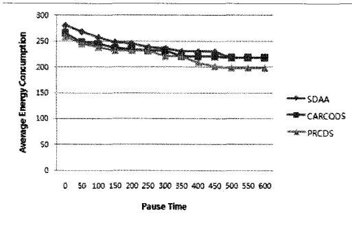
그림 13. 노드 이동성에 따른 에너지 소비
