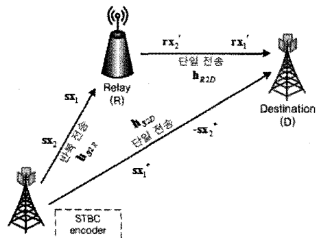
그림 2. 제안하는 협력 통신 방법
