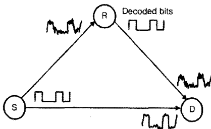
그림 1. 복호 후 전송 협력 통신 방법
