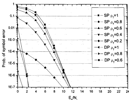
그림 9. 펄스 재밍 환경에서 Link-16의 심볼 에러 확률 ( E_b/N_0=10\text{dB} , Link-16 시스템 요소 고려)
