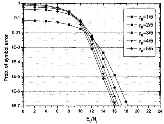
그림 6. 부분대역 잡음 재밍 환경에서 Link-16의 심볼 에러 확률( E_b/N_0=10 dB, single-pulse)
