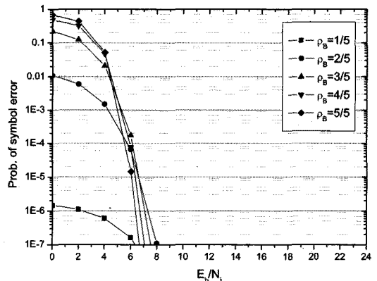
그림 7. 부분대역 잡음 재밍 환경에서 Link-16의 심볼 에러 확률( E_b/N_0=10 dB, double-pulse)
