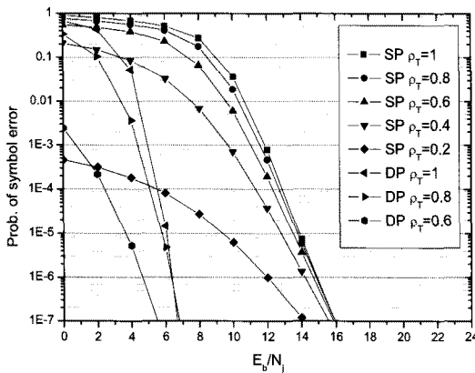
그림 8. 펄스 재밍 환경에서 Link-16의 심볼 에러 확률 ( E_b/N_0=10\text{dB} )
