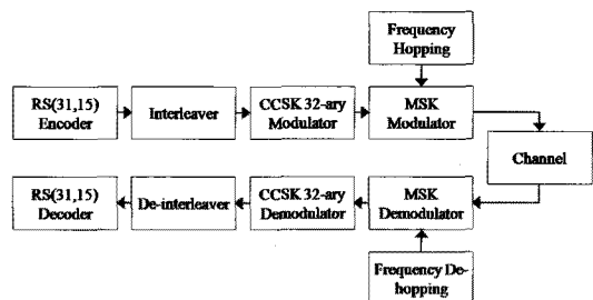
그림 1. JTIDS 송수신 모델
