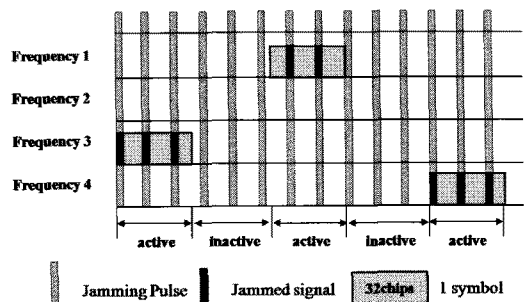
그림 4. 펄스 재밍
