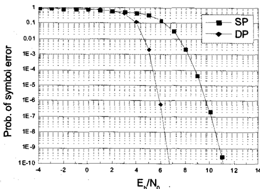
그림 5. 재밍이 없을 경우 Link-16의 심볼 에러 확률 (single-pulse, double-pulse)
