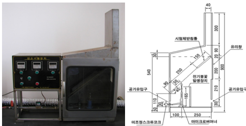
[그림 4] 연소시험장치
