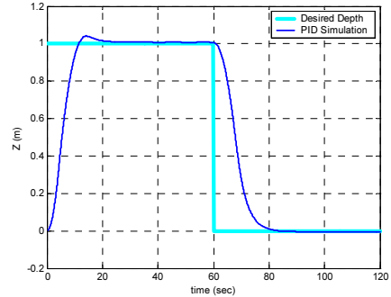
[그림 11] Simulation result of depth control
