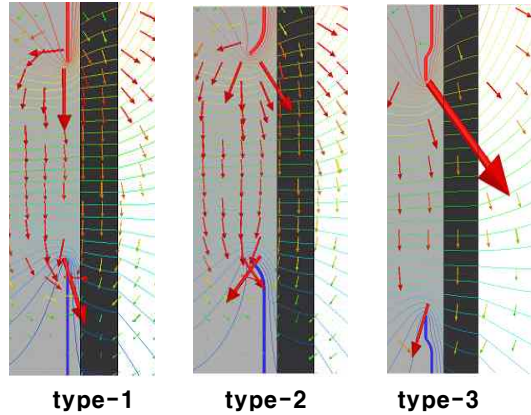
그림 4. 전계분포 및 등전위분포. Fig. 4. E field and potential line of each model.
