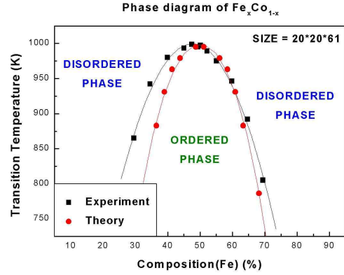
그림 2. FeCo 합금의 상도표. Fig. 2. Phase diagram of FeCo alloy.
