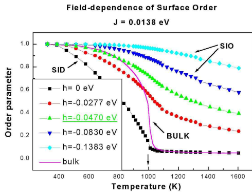
그림 3. 장의 세기에 따른 표면 질서도. Fig. 3. Filed dependence of surface order.
