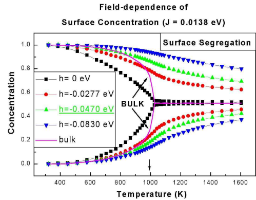
그림 4. 장의 세기에 따른 표면 편석. Fig. 4. Filed dependence of surface segregation.
