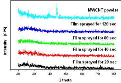
그림 3. 스프레이 시간에 따른 MWCNT막의 XRD 패턴. Fig. 3. XRD patterns of MWCNT films with the various spray time.
