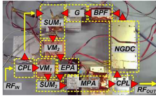
그림 12. NGDC를 이용한 아날로그 피드백 구조의 제작 사진
