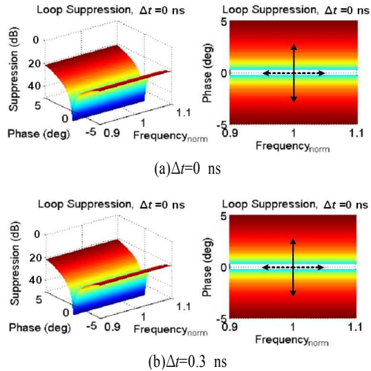
그림 3. \Delta V=0.01 dB일 때 위상 및 균지연 부정합에 대하여 표현한 루프 상쇄도 [23]
