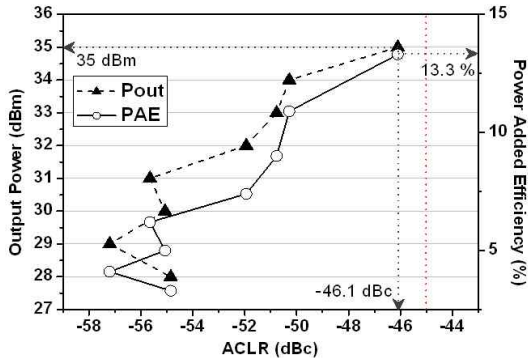
그림 11. 1-carrier WCDMA 신호에 대한 ACLR 및 PAE 상관 관계
