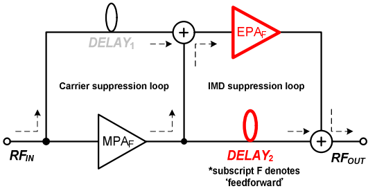
(a) 일반적인 피드포워드 증폭기 (a) The typical feedforward amplifier
