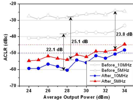
그림 10. 10 dB 출력 동적 영역에 대한 5 MHz, 10 MHz 이격된 주파수에서 선형화 전/후의 ACLR 특성
