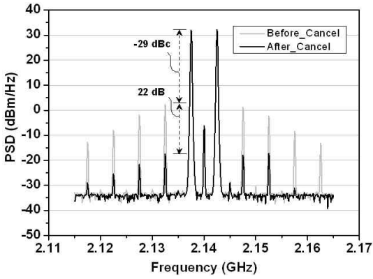
그림 8. 32 dBm/ton의 출력 전력에서 측정된 선형화 전/후의 2-tone 스펙트럼
