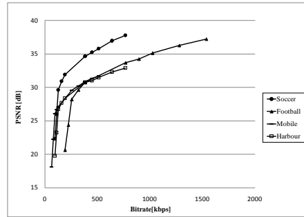
Fig. 4. SVC R-D curves
