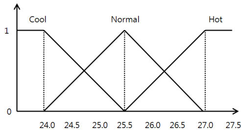
그림 3. 온도 값에 대한 소속 함수 Fig. 3. Membership functions for Temperature
