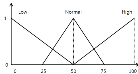
그림 4. 습도에 대한 소속 함수 Fig. 4. Membership function for humidity
