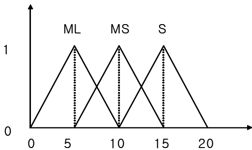
그림 5. 풍속에 대한 소속 함수 Fig. 5. Membership functions for wind speed
