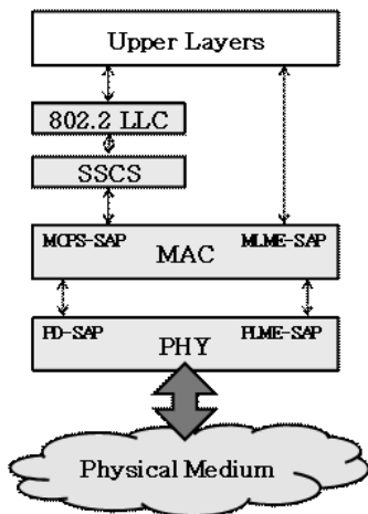
(그림 1) LR-WPAN 디바이스 구조
