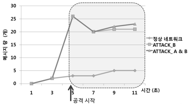
(그림 10) 공격 후 Beacon Request 전송 메시지 수
