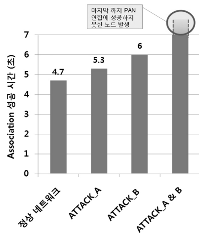
(그림 12) 모든 노드 Association 완료 시간
