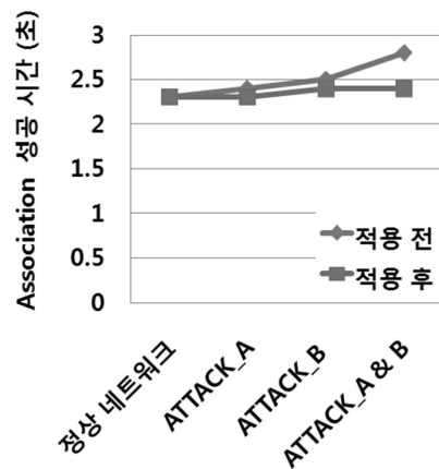
(그림 13) 탐지 메커니즘 적용 후, 노드의 Association 평균 시간 비교
