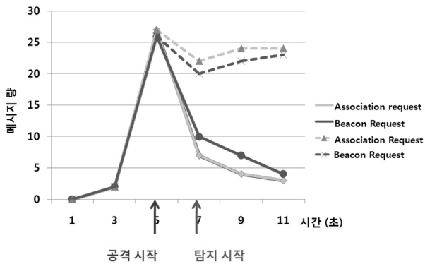
(그림 19) 공격과 탐지 메커니즘에 따른 메시지 변화량
