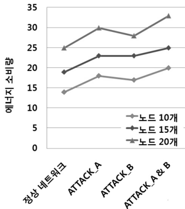
(그림 17) 노드량에 따른 코디네이터 에너지소모량
