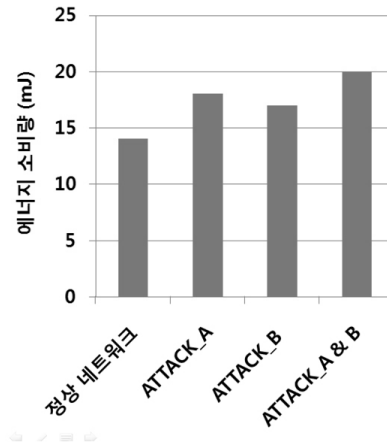
(그림 16) 코디네이터의 에너지소모량
