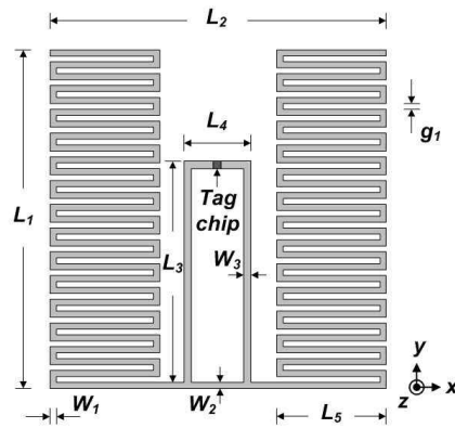
그림 1. 제안된 태그 안테나 구조(20×19.7 mm 2 ) Fig. 1. Structure of the proposed tag antenna(20×19.7 mm 2 ).
