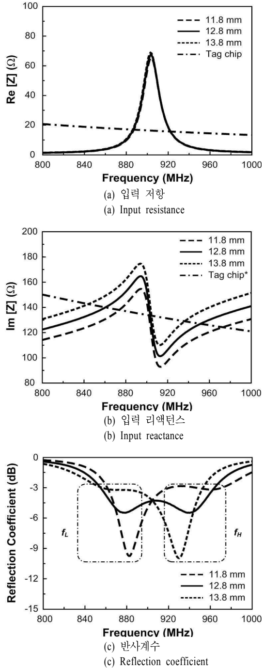
그림 2. 사각 형태의 급전부 상하 길이( L_3 ) 변화에 따른 특성 변화 Fig. 2. Variation of antenna characteristic with respect to the vertical length( L_3 ) of the feed line.
