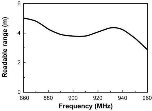
그림 6. 주파수에 따른 최적화된 태그 안테나 인식 거리 특성
