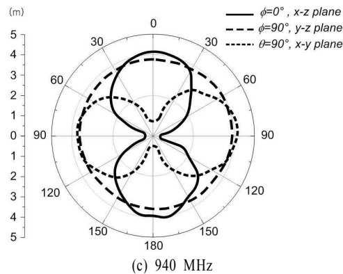
그림 7. 방향에 따른 최적화된 태그 안테나 인식 거리 특성
