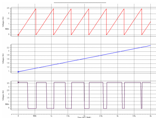
Fig. 17. Simulation result of comparator 그림 17. 비교기 시뮬레이션
