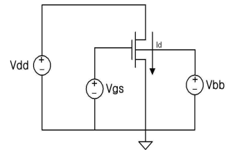
Fig. 5. Switching characteristic simulation circuit 그림 5. Switching 특성 시뮬레이션 회로
