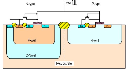
Fig. 4. The design of DT-CMOS in Bulk CMOS 그림 4. Bulk CMOS에서의 DT-CMOS 구현
