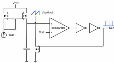
Fig. 15. saw tooth wave generator 그림 15. 삼각파 발생기
