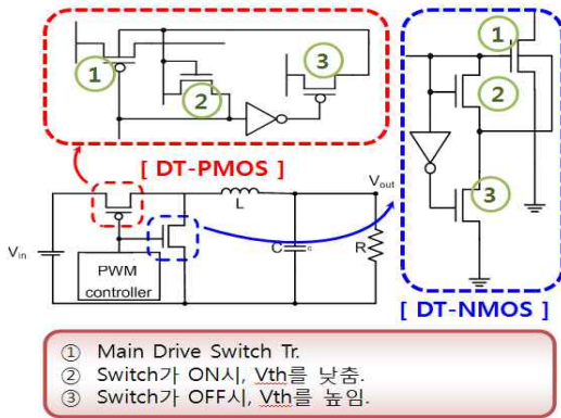
Fig. 3. Leakage current control method in DTMOS 그림 3. DTMOS에서 누설전류 제어기법
