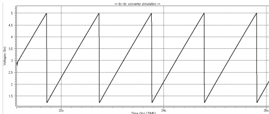
Fig. 16. Simulation result of saw tooth wave generator 그림 16. 삼각파 발생기 시뮬레이션
