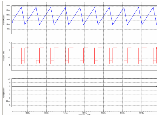
Fig. 18. Simulation result of DC-DC converter 그림 18. DC-DC converter의 시뮬레이션 결과
