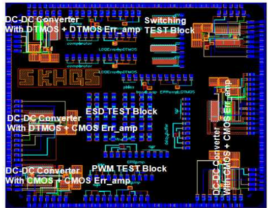
Fig. 22. Layout of DC-DC converter 그림 22. DC-DC 컨버터 배치도
